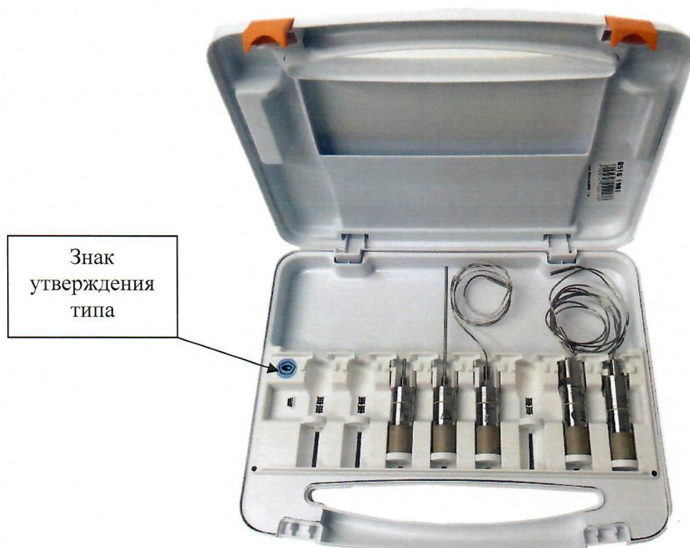
Рисунок 2 - Общий вид блока считывания и конфигурации с уложенными в нем регистраторами беспроводными Testo 190 и место нанесения знака утверждения типа
