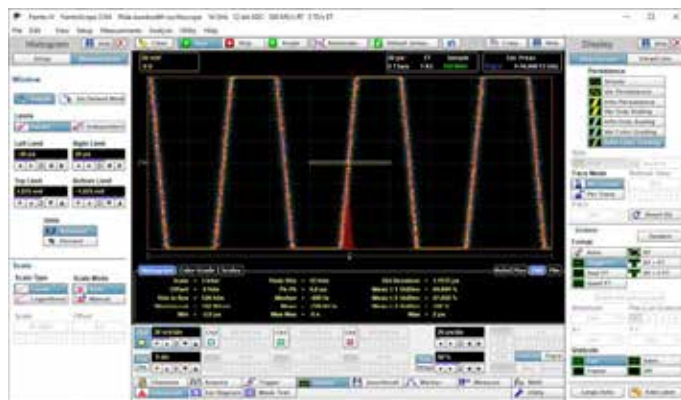
Рис. 14 Синхронизация сигнала синусоидальной формы частотой 16 ГГц осциллографом АКПП-4139/2, джиттер синхронизации 1,11 пс
