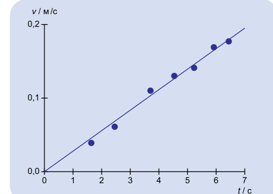
Рис. 3. График скорости в зависимости от времени для начального движения вниз
