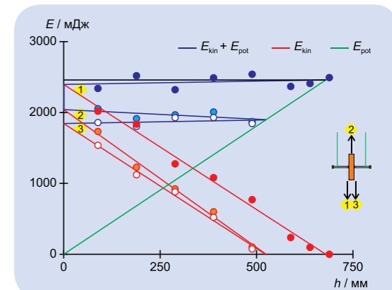
Рис. 4. Распределение энергии как функция высоты h
