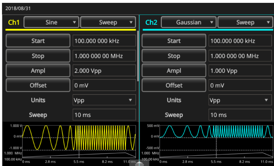
Рисунок 35: Настройки сигнала в режиме свипирования
