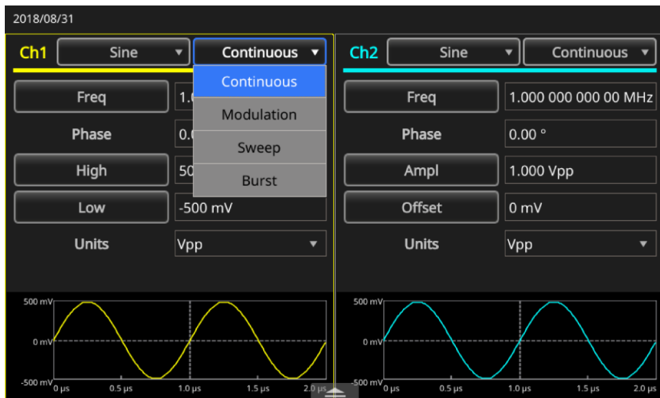
Рисунок 11: Выбор непрерывного режима работы
