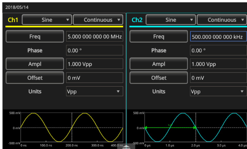
Рисунок 152: Настройка формы сигнала
