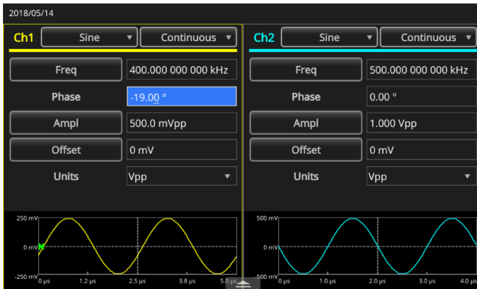
Рисунок 155: Изменение фазы сигнала K1 на -19^\circ
