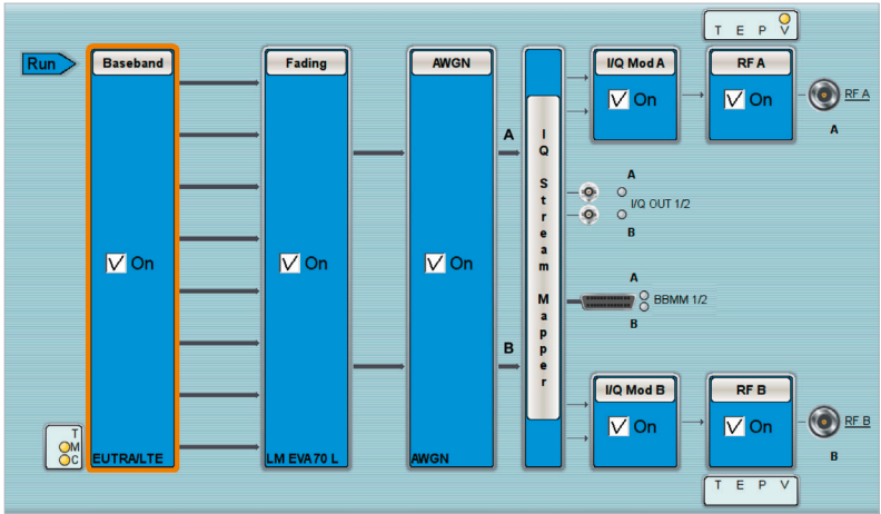
Пример конфигурации 3: Генератор R&S®SMW200A в максимальной комплектации с опцией MIMO поддерживает все основные сценарии MIMO, включая вариант 8x2, показанный на данном снимке экрана. В данном случае секция модулирующего сигнала имеет восемь источников сигнала и 32 логических канала с замираниями (каналы MIMO).
