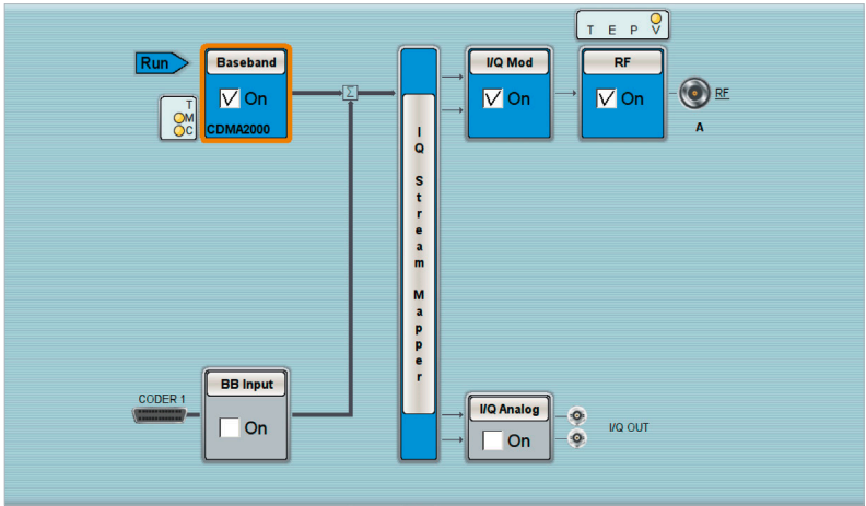
Пример конфигурации 1: Одноканальный генератор R&S®SMW200A со встроенным генератором модулирующего сигнала можно использовать для измерения отдельных компонентов или для базовых испытаний приемника.
