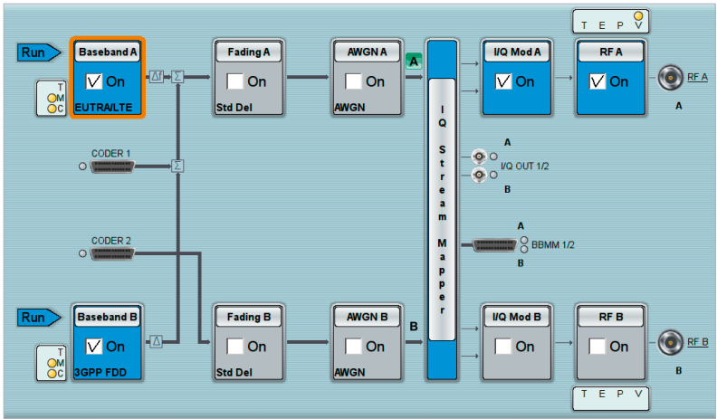
Пример конфигурации 2: Двухканальный генератор R&S®SMW200A идеально подходит для испытаний приемников и характеристик базовых станций. Один генератор может формировать сумму полезного сигнала и помехи (в данном примере полезный сигнал LTE и помеха 3GPP FDD).
