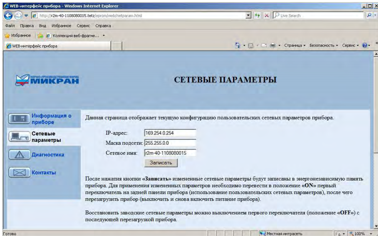
Рисунок 3.5 – Изменение сетевых параметров
