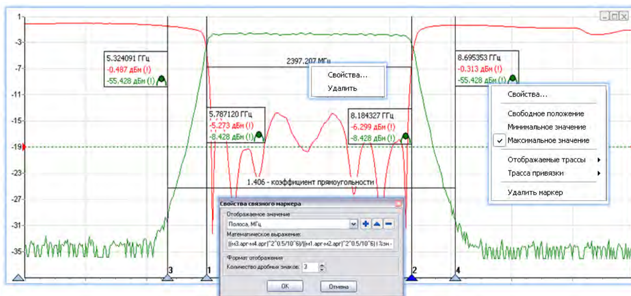
Рисунок 3.42 – Использование маркеров
