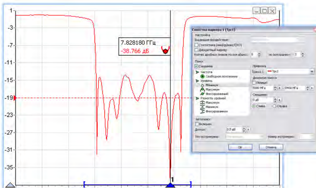
Рисунок 3.44 – Следящий маркер
