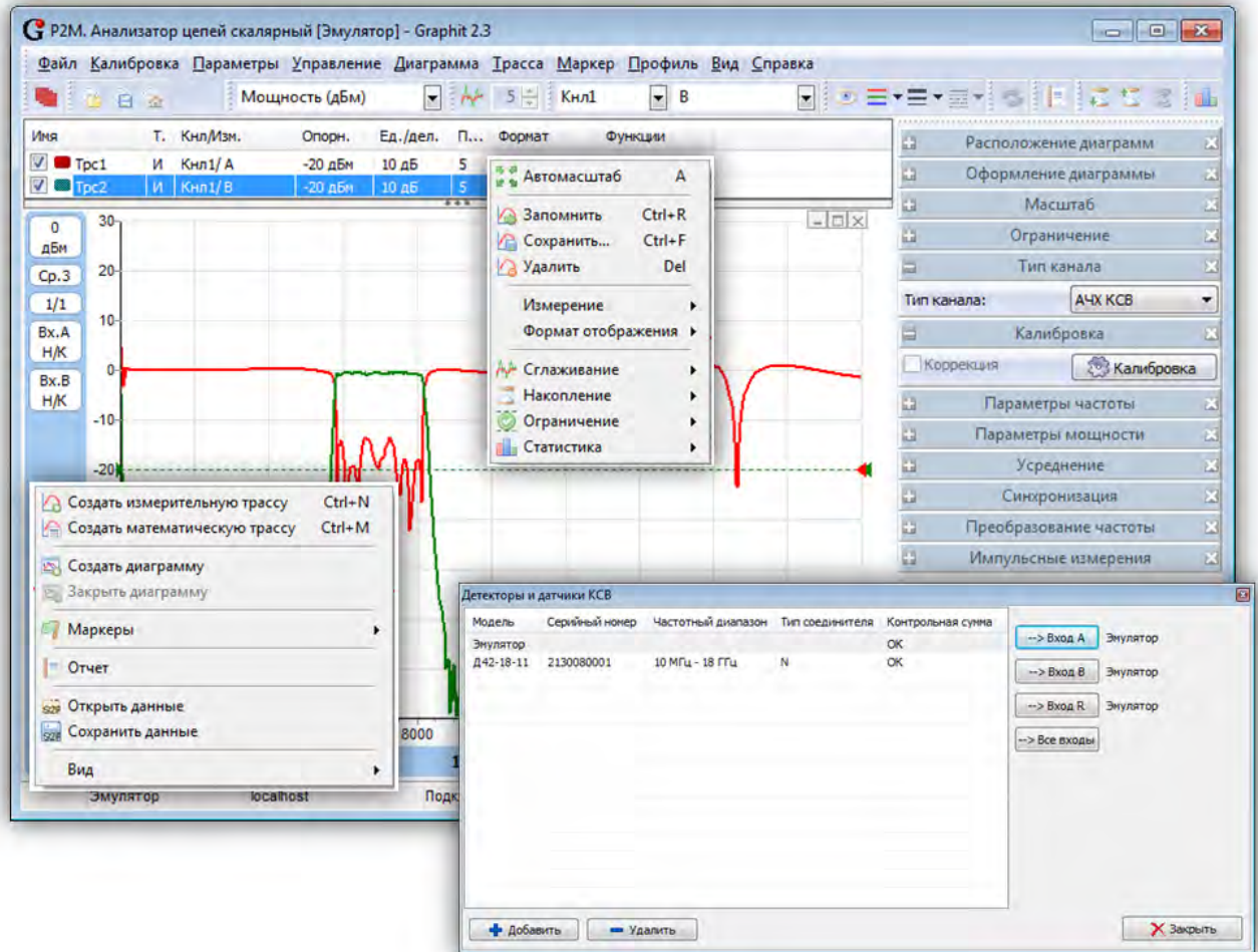
Рисунок 21 – Программное обеспечение
