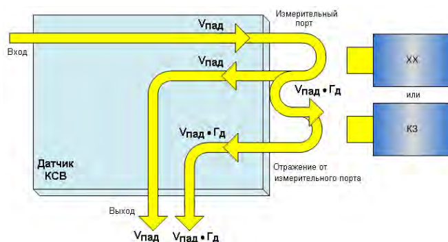
Рисунок 22 – Паразитное отражение от измерительного порта датчика КСВ (после нормировки на напряжение падающей волны V_{\text{пад}} : 1 \pm \Gamma_d , где \Gamma_d – модуль коэффициента отражения измерительного порта датчика КСВ)
