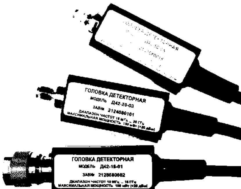
Рисунок 17 – Головки детекторные
