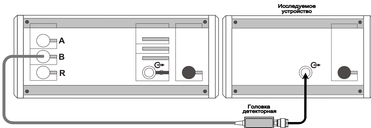
Рисунок 5.5 – Схема измерений мощности на выходе устройств со встроенными источниками сигналов
