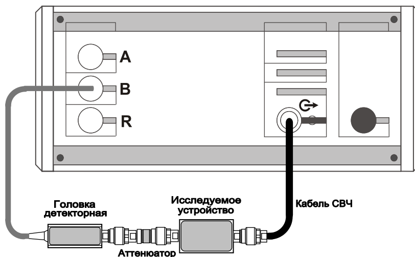
Рисунок 5.26 – Типичная схема измерения динамических характеристик
