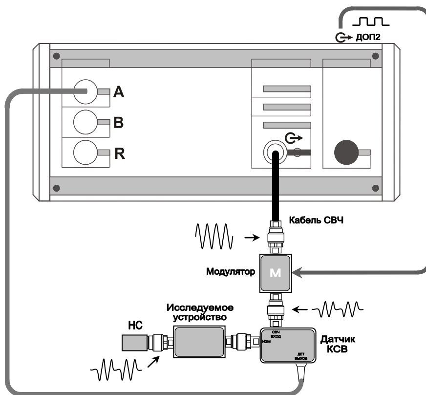
Рисунок 5.36 – Схема измерения модуля КО с внутренним синхрогенератором
