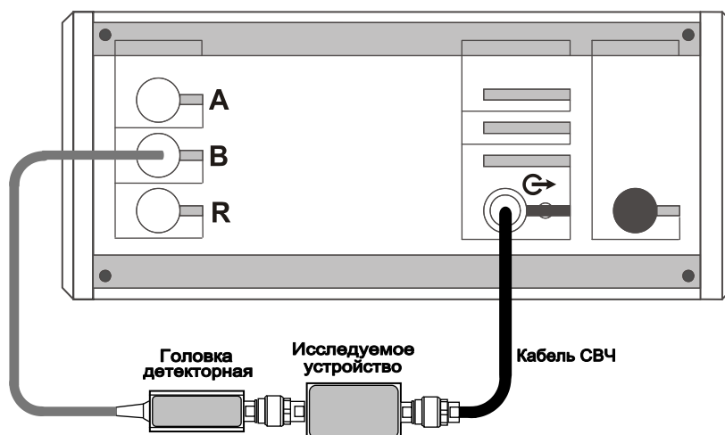
Рисунок 5.6 – Схема измерений мощности на выходе ИУ с внешним сигналом
