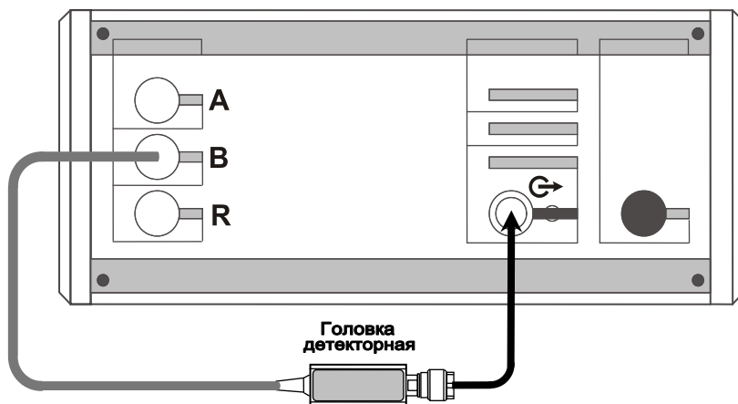
Рисунок 5.41 – Схема калибровки КП с внешним синхрогенератором
