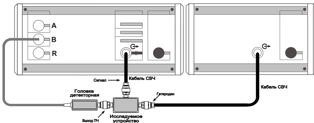
Рисунок 5.15 – Измерение с фиксированной частотой гетеродина
