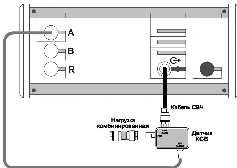
Рисунок 5.39 – Схема калибровки КО
