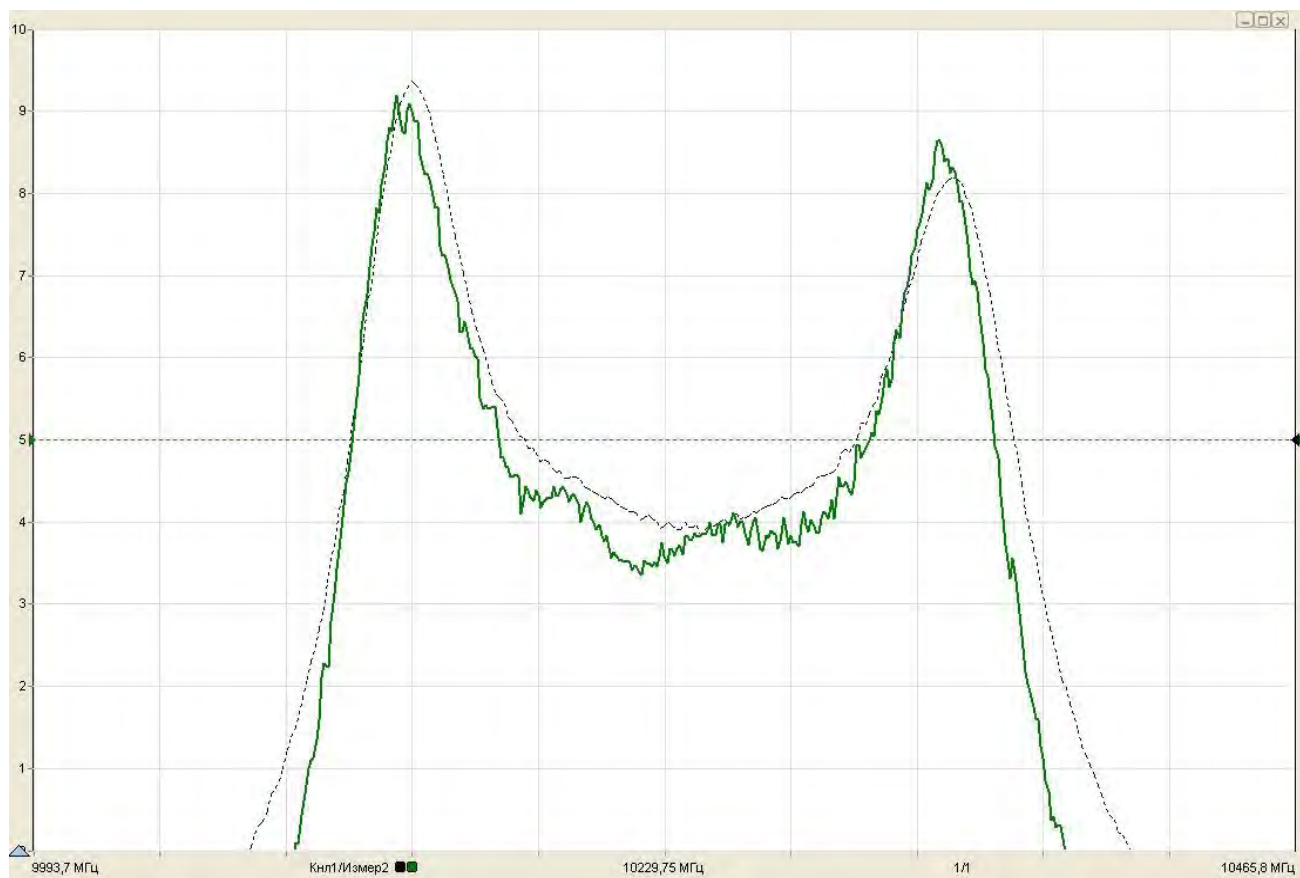
Рисунок 5.33 – Результаты измерений ГВЗ
