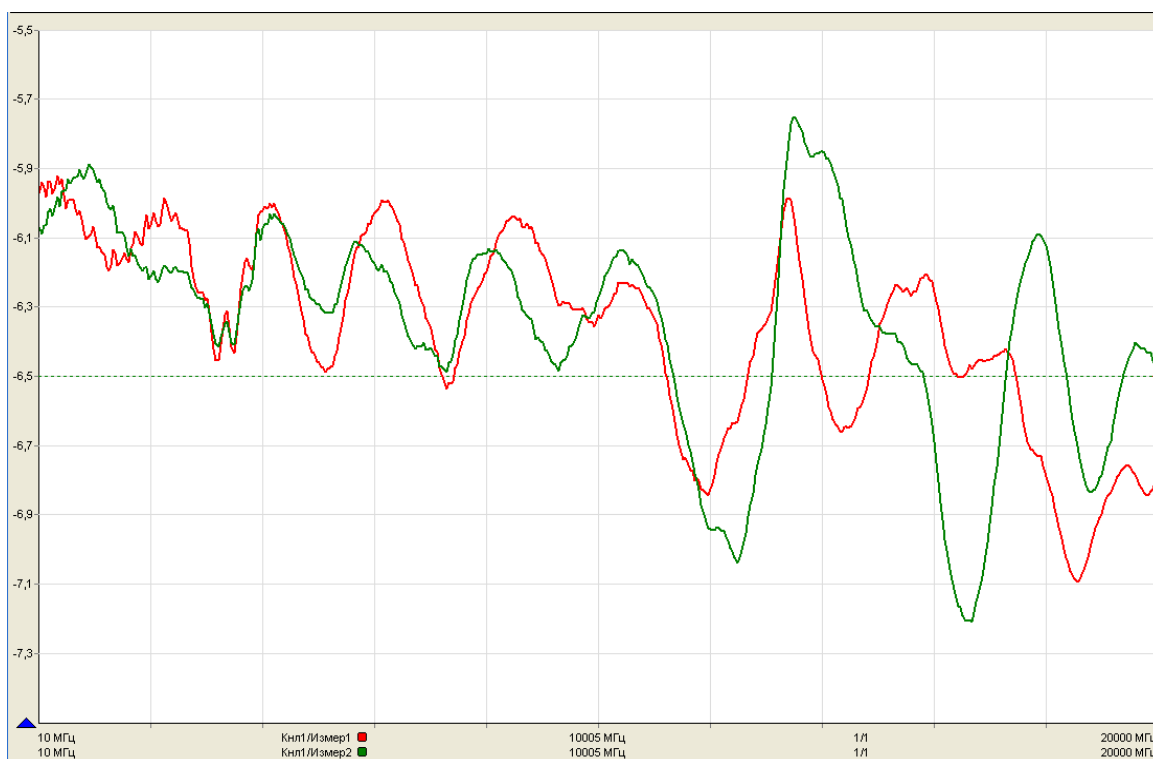
Рисунок 5.13 – Графики измерения модулей КП делителя мощности
