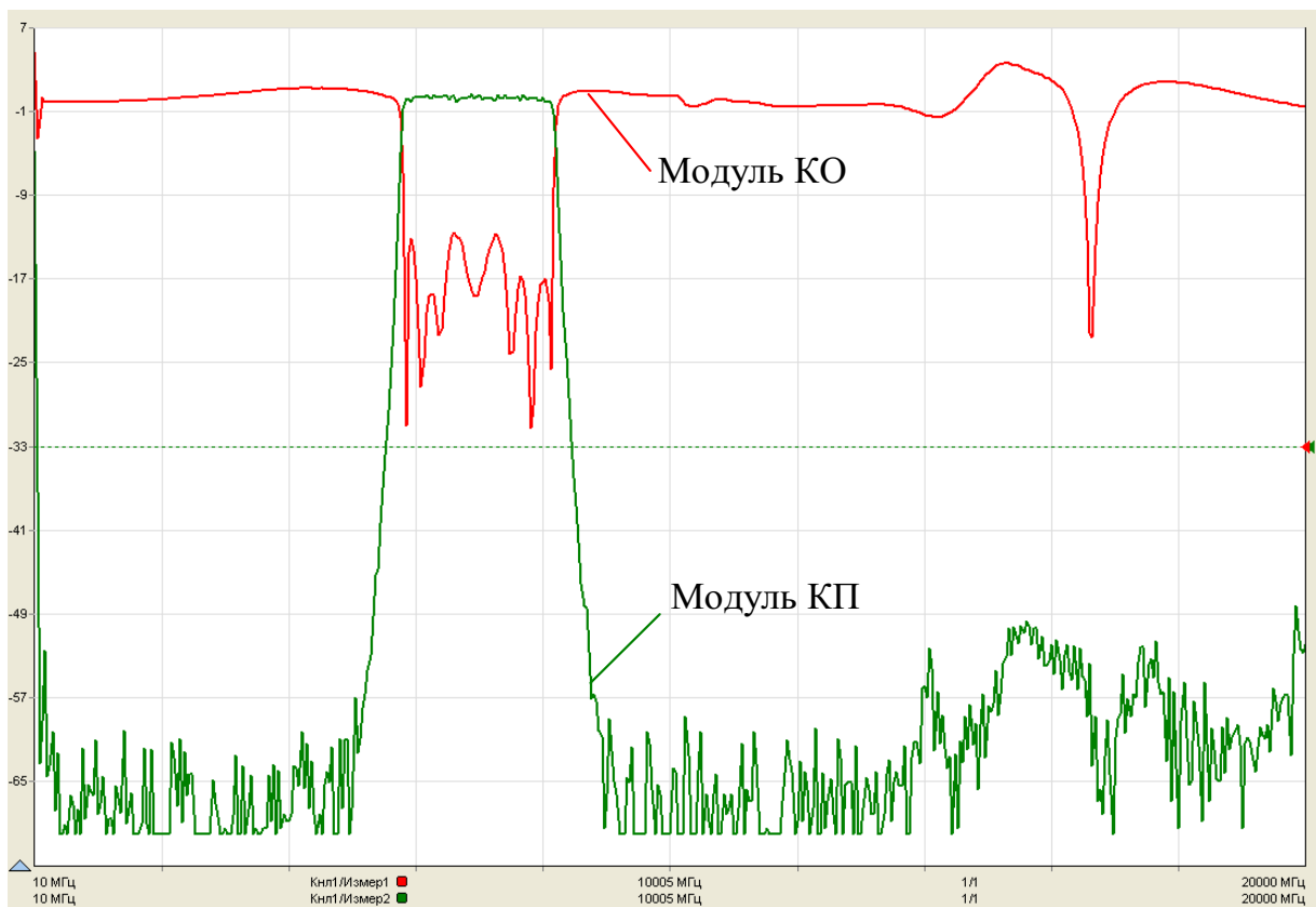
Рисунок 5.25 – Результаты одновременных измерений модулей КП и КО полосового фильтра
