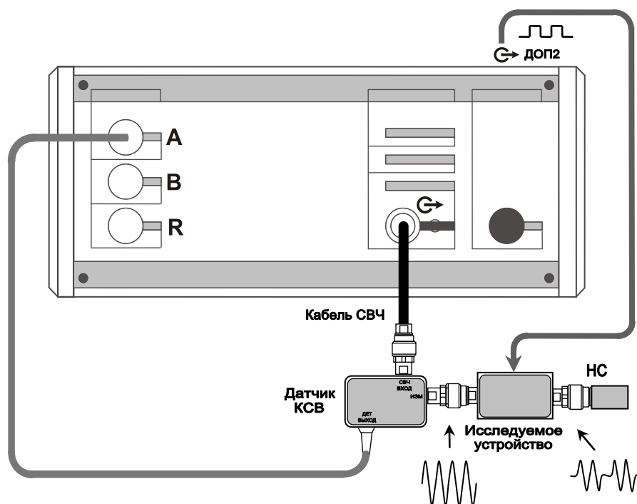
Рисунок 5.40 – Схема измерения модуля КО с внутренним синхрогенератором
