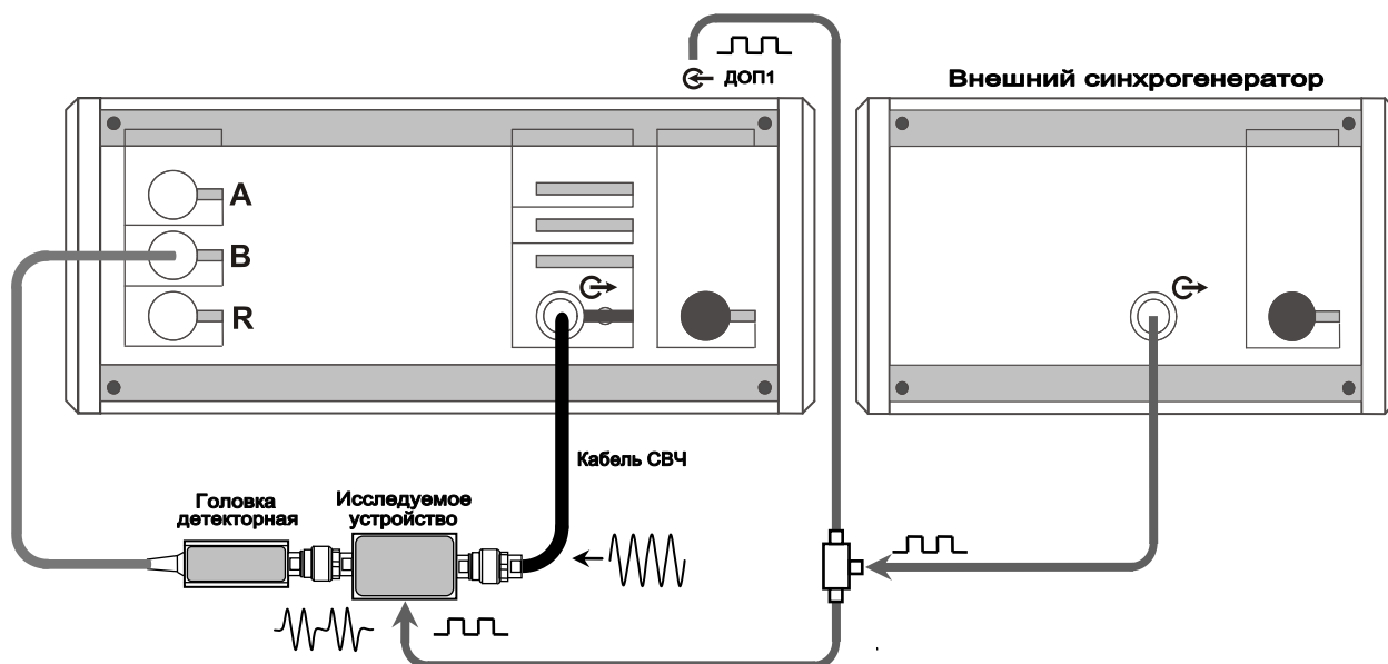
Рисунок 5.42 – Схема измерения модуля КП с внешним синхрогенератором
