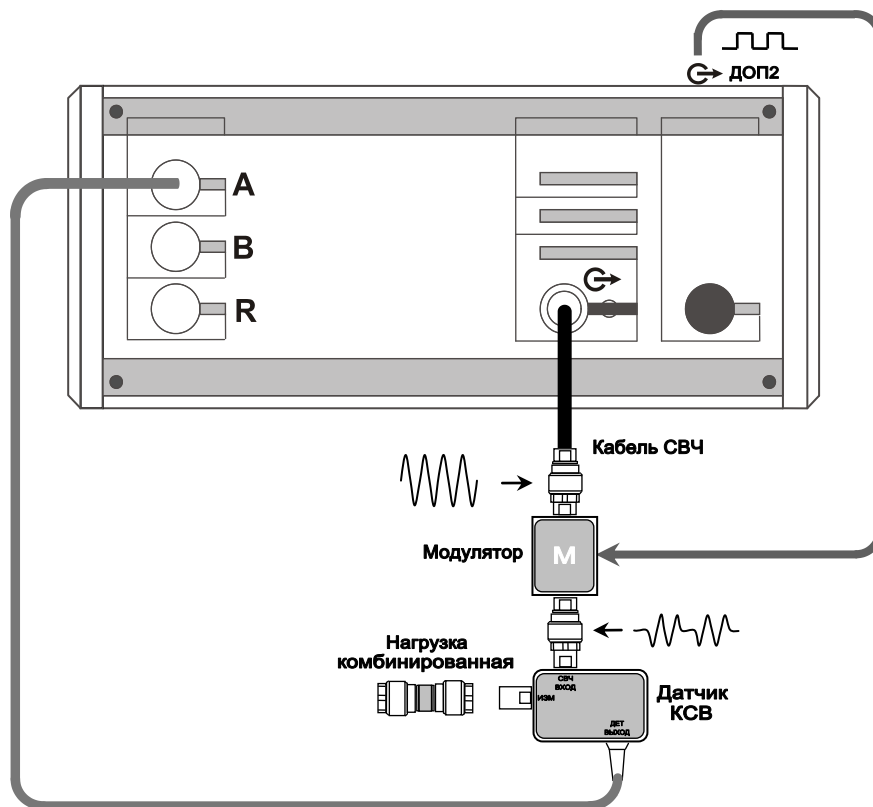
Рисунок 5.35 – Схема калибровки КО с внутренним синхрогенератором
