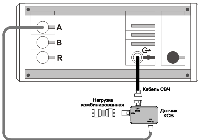
Рисунок 5.17 – Схема калибровки в режиме измерений модуля КО, КСВН
