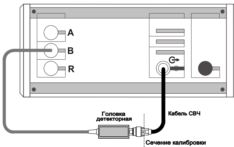
Рисунок 5.8 – Схема калибровки в режиме измерений модуля КП
