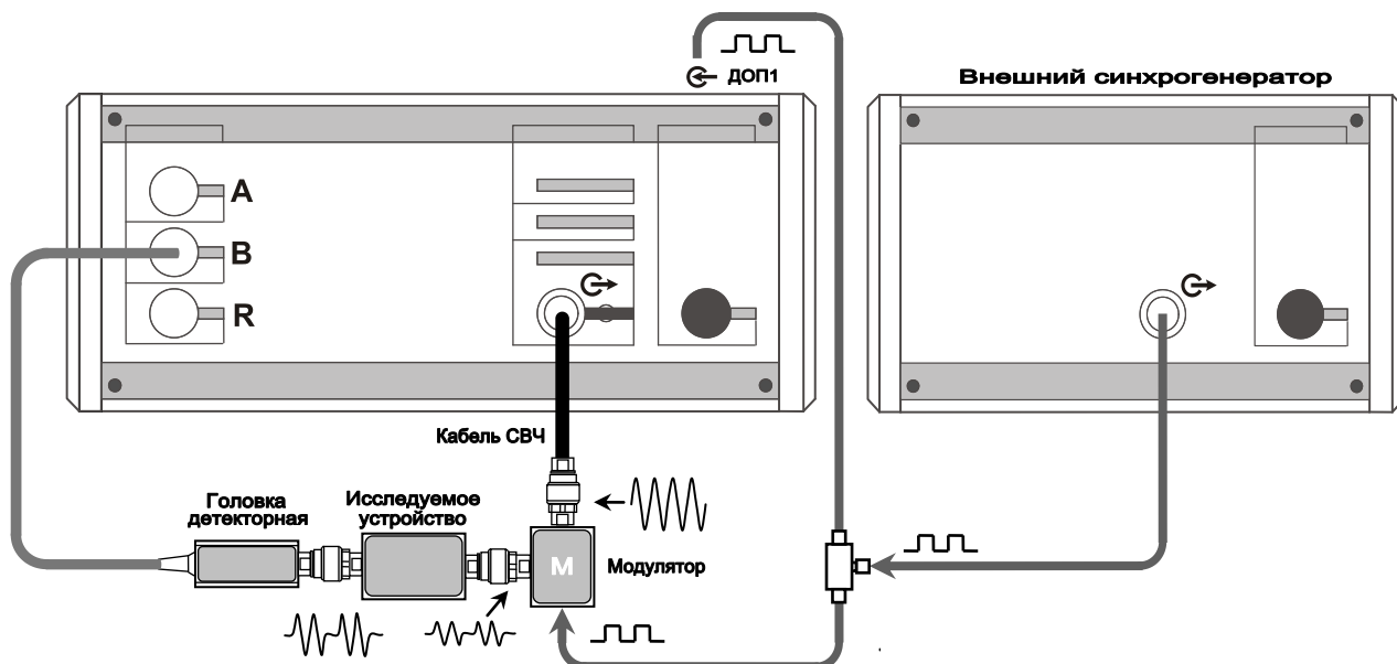
Рисунок 5.38 – Схема измерения модуля КП с внешним синхрогенератором
