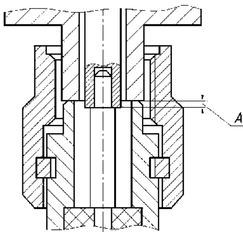
Рисунок 4.7 – Проверка размера «А» соединителя «вилка» для соединителей типов IX вариант 3 и 3,5 мм
