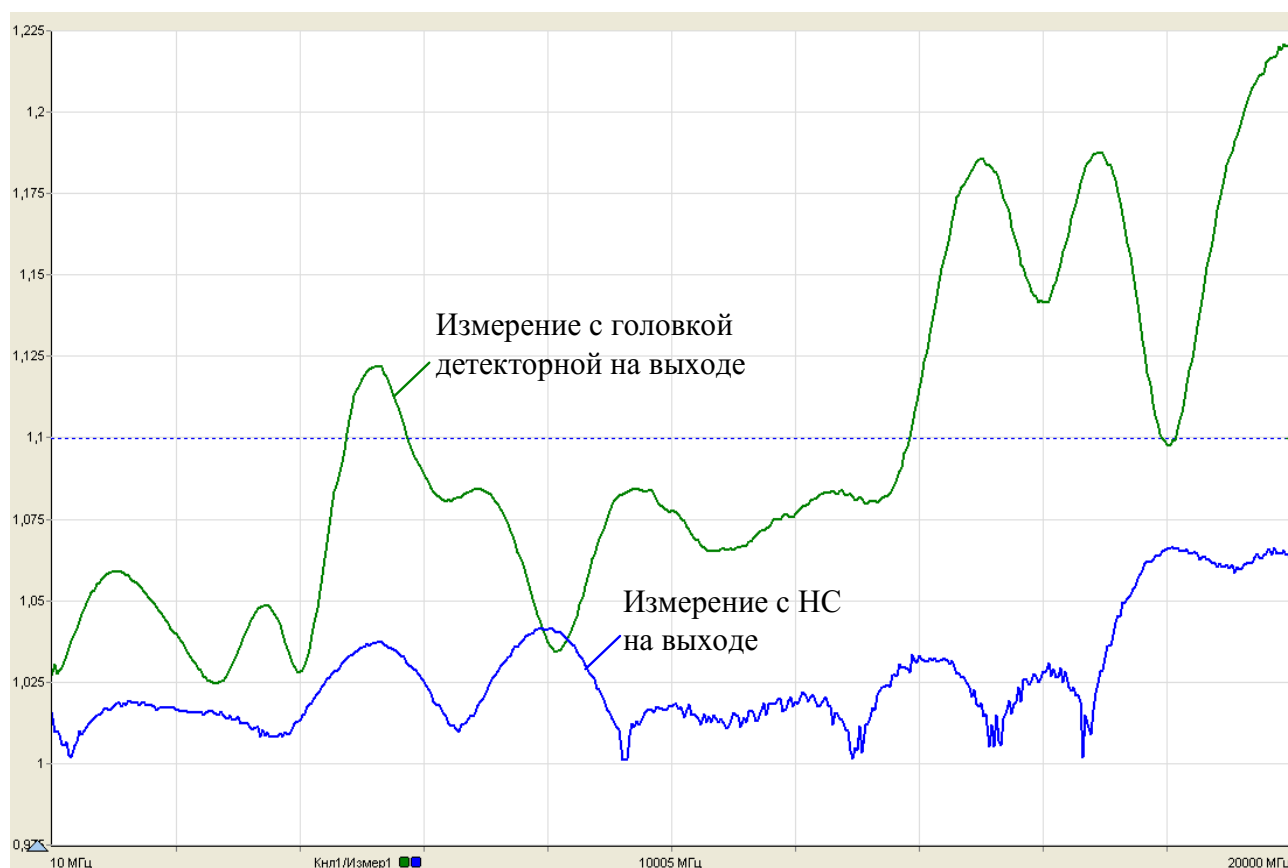
Рисунок 5.21 – Результаты измерений КСВН перехода
