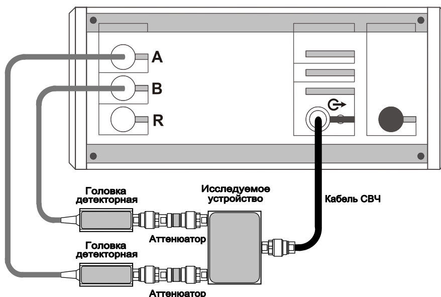
Рисунок 5.12 – Схема измерений модуля КП трехпортовых устройств без преобразования частоты
