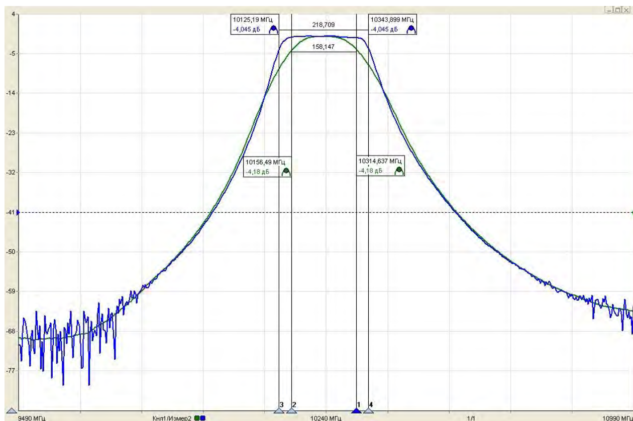
Рисунок 5.9 – График измерения модуля КП полосового фильтра
