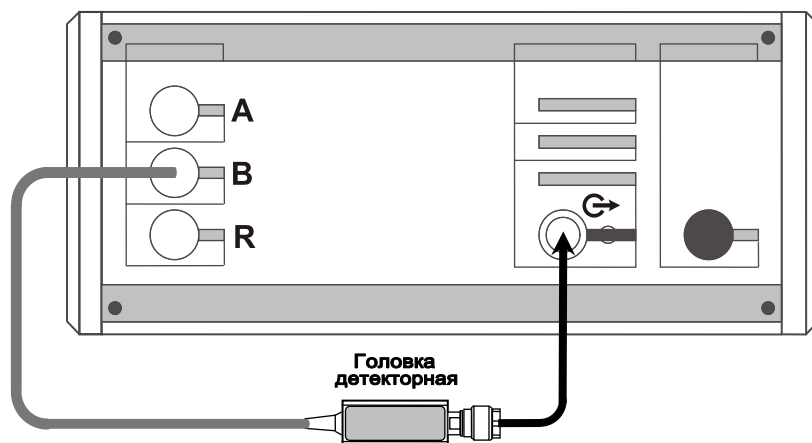
Рисунок 5.32 – Схема калибровки в режиме измерений модуля КП п) запустить мастер калибровки измерительной трассы для входа «В» в
