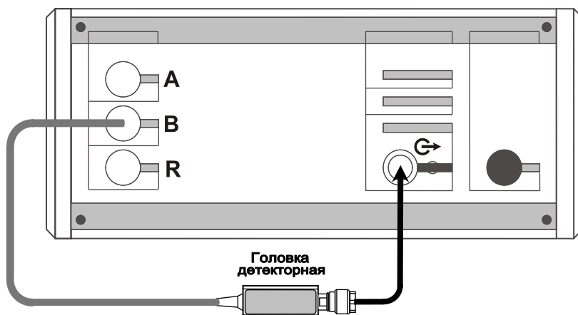
Рисунок 4.10 – Схема измерений мощности
