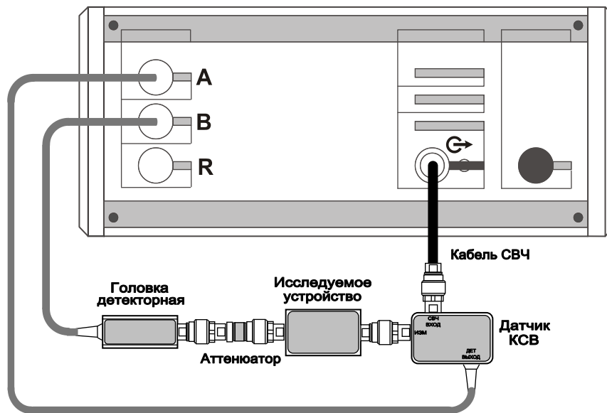
Рисунок 5.24 – Типичная схема измерений модуля КП и КО
