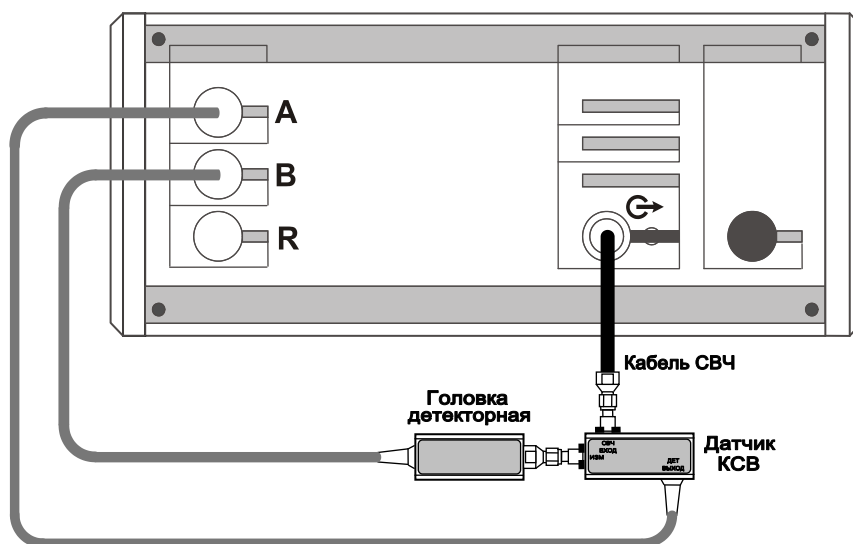
Рисунок 4.9 – Схема калибровки в режиме одновременного измерения модуля КП и модуля КО: а) в тракте 7,0/3,04; б) в тракте 3,5/1,52.
