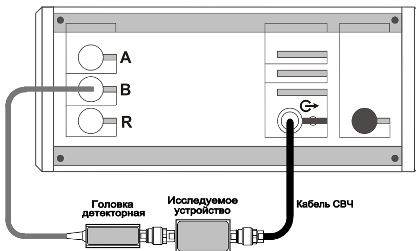
Рисунок 5.7 – Схема измерений модуля КП двухпортовых устройств
