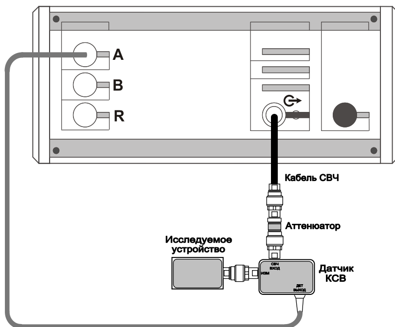
Рисунок 5.16 – Схема измерения модуля КО с согласующим аттенюатором
