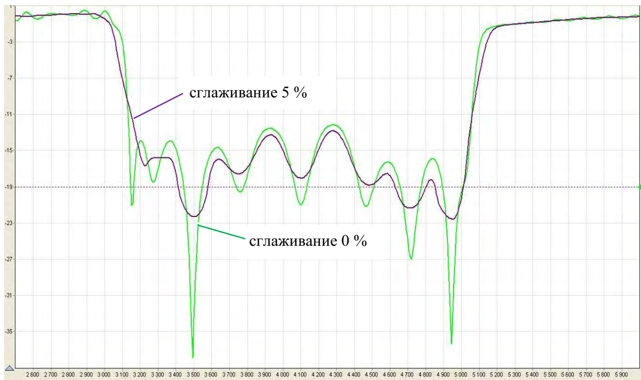
Рисунок 5.20 – Результаты измерений модуля КО полосового фильтра при разных уровнях сглаживания (в децибелах)
