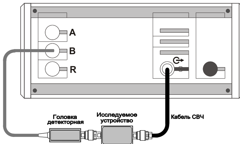
Рисунок 5.31 – Схема измерений
