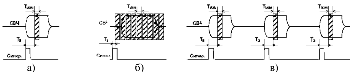
Рисунок 5.34 – Варианты выборки импульса
