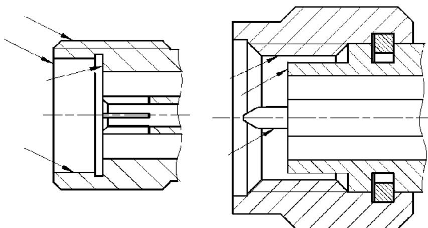
Рисунок 4.2 – Очищаемые поверхности коаксиальных соединителей типов IX вар.3 и 3,5 мм
