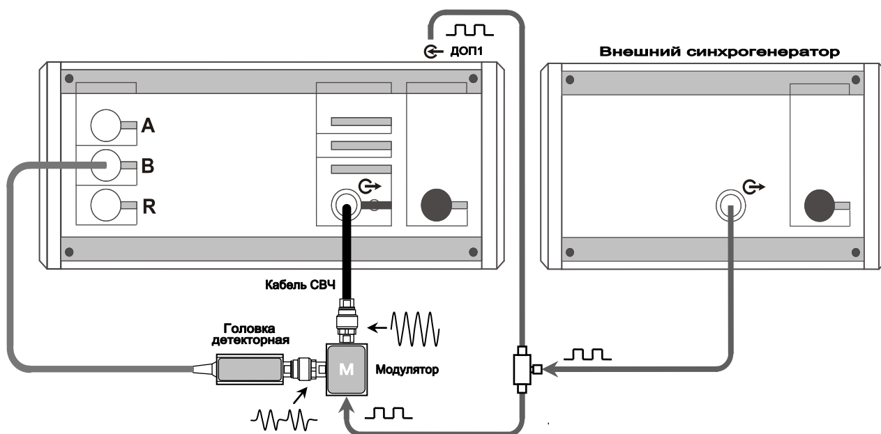
Рисунок 5.37 – Схема калибровки КП с внешним синхрогенератором
