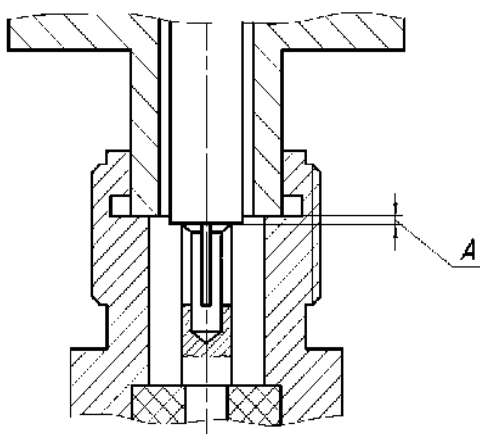
Рисунок 4.5 – Проверка размера «А» соединителя «розетка» для соединителей типов IX вариант 3 и 3,5 мм
