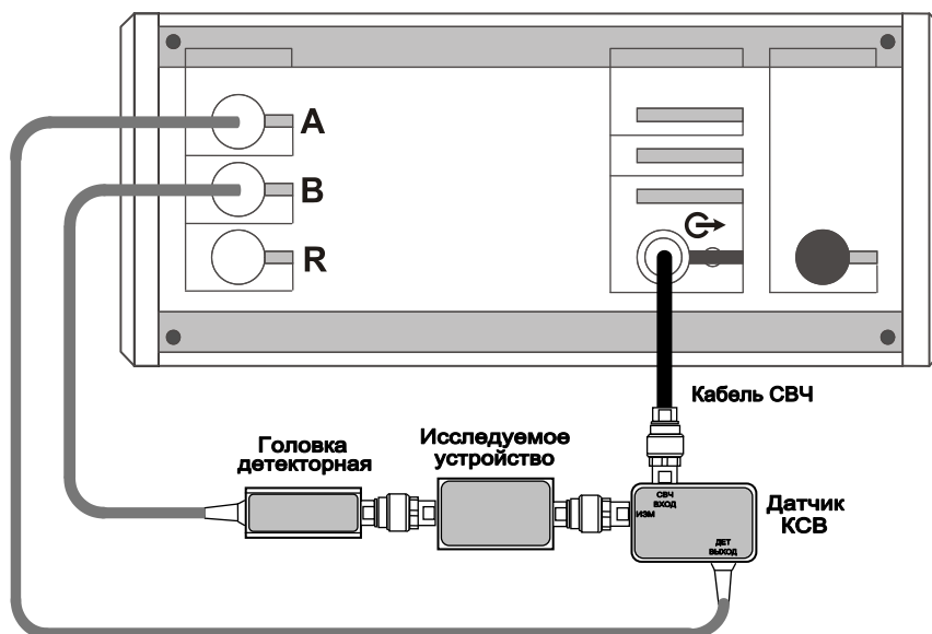
Рисунок 5.23 – Типичная схема измерений модуля КП и КО
