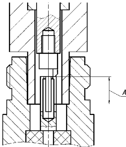
Рисунок 4.4 – Проверка размера «А» соединителя «розетка» для соединителей типов III и N
