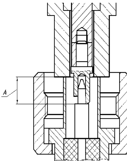
Рисунок 4.6– Проверка размера «А» соединителя «вилка» для соединителей типов III и N
