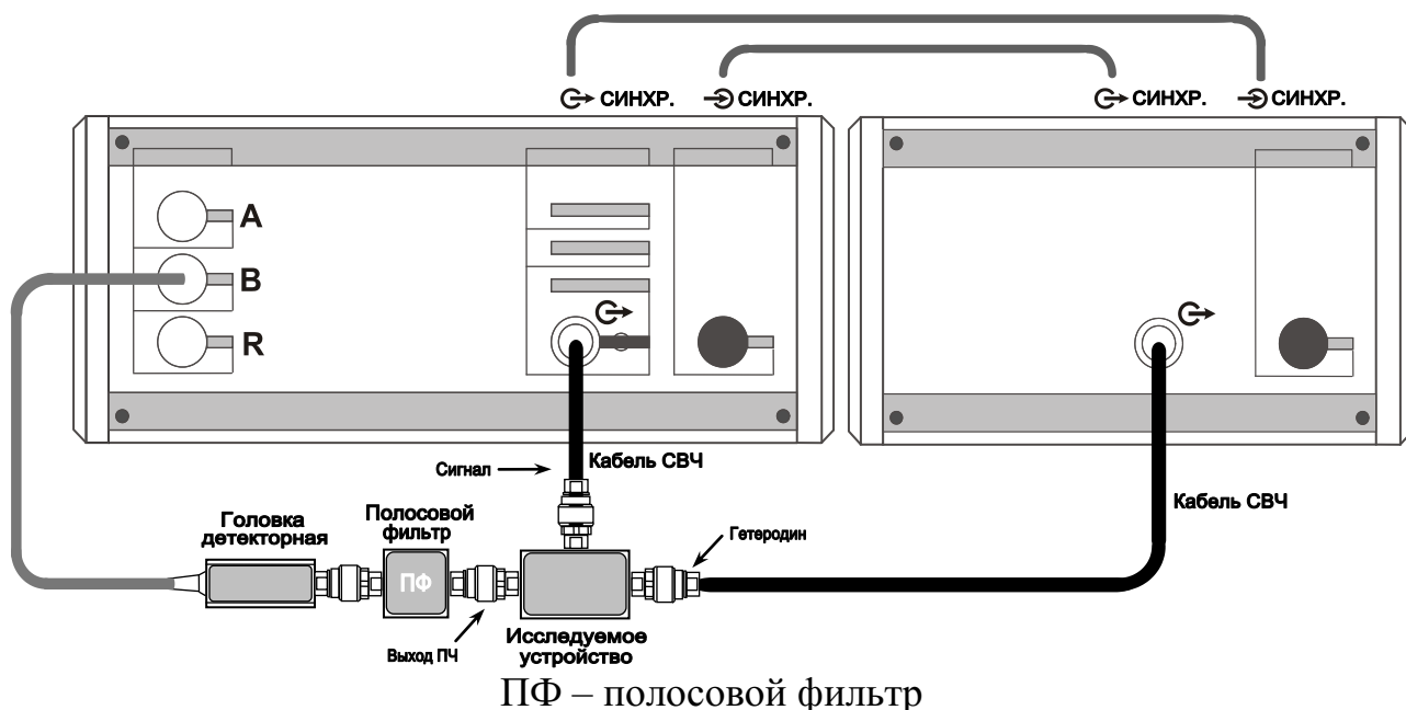
Рисунок 5.14 – Синхронная перестройка частоты сигнала и гетеродина
