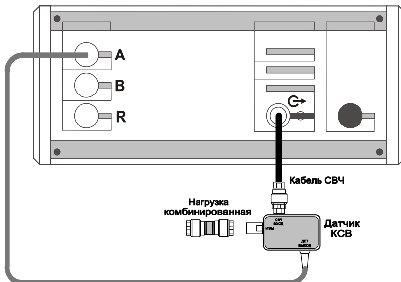
Рисунок 4.8 – Схема калибровки в режиме измерений модуля КО
