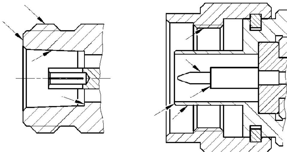
Рисунок 4.1 – Очищаемые поверхности коаксиальных соединителей типов III и N
