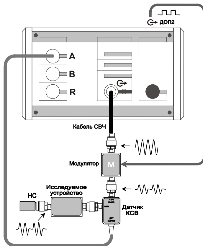
Рисунок 5.35 – Схема измерения модуля КО с внутренним синхрогенератором
