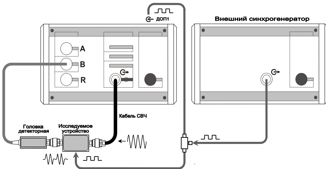
Рисунок 5.41 – Схема измерения модуля КП с внешним синхрогенератором
