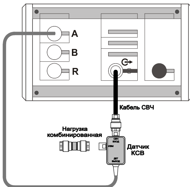
Рисунок 5.16 – Схема калибровки в режиме измерений модуля КО, КСВН
