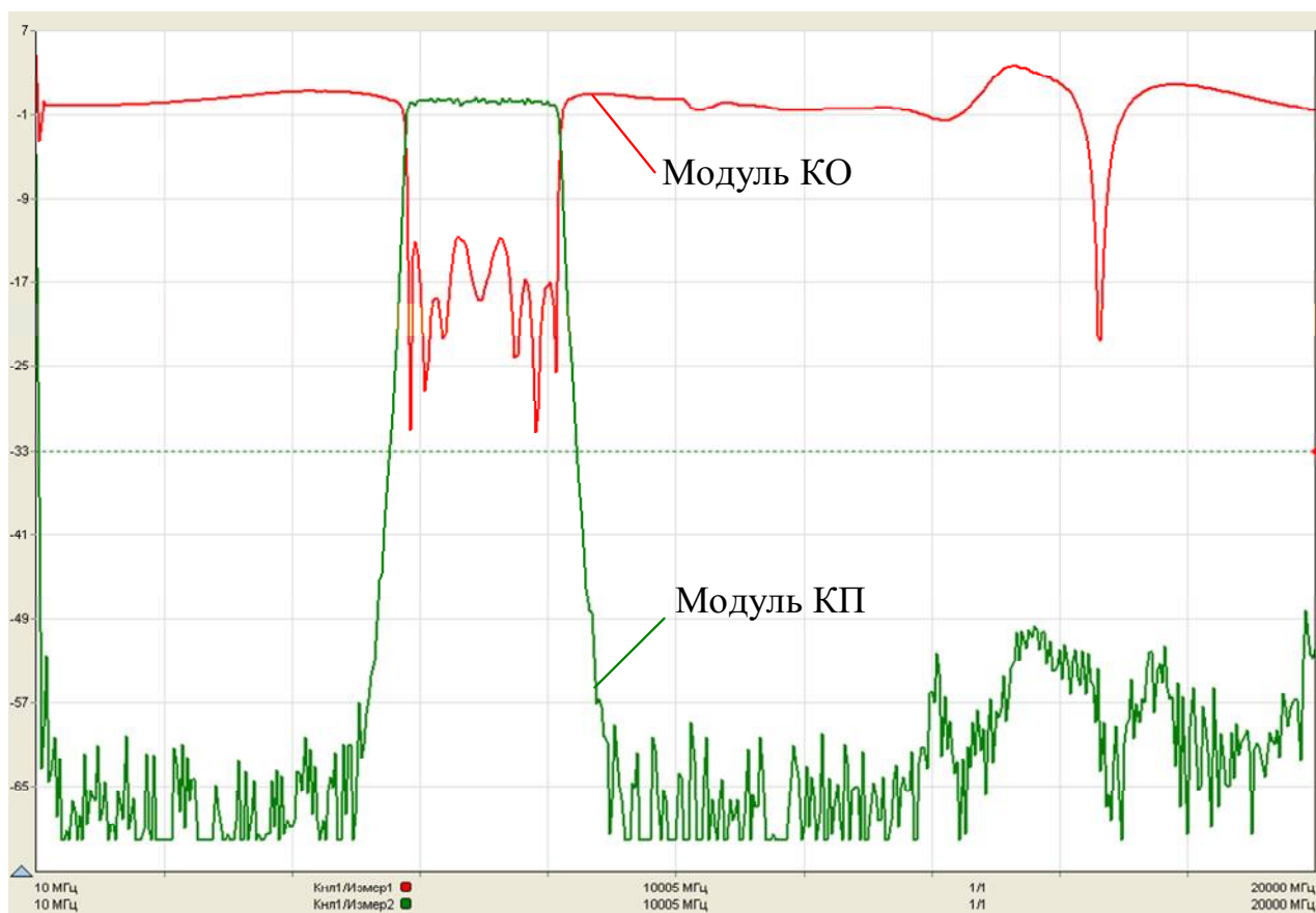
Рисунок 5.24 – Результаты одновременных измерений модулей КП и КО полосового фильтра
