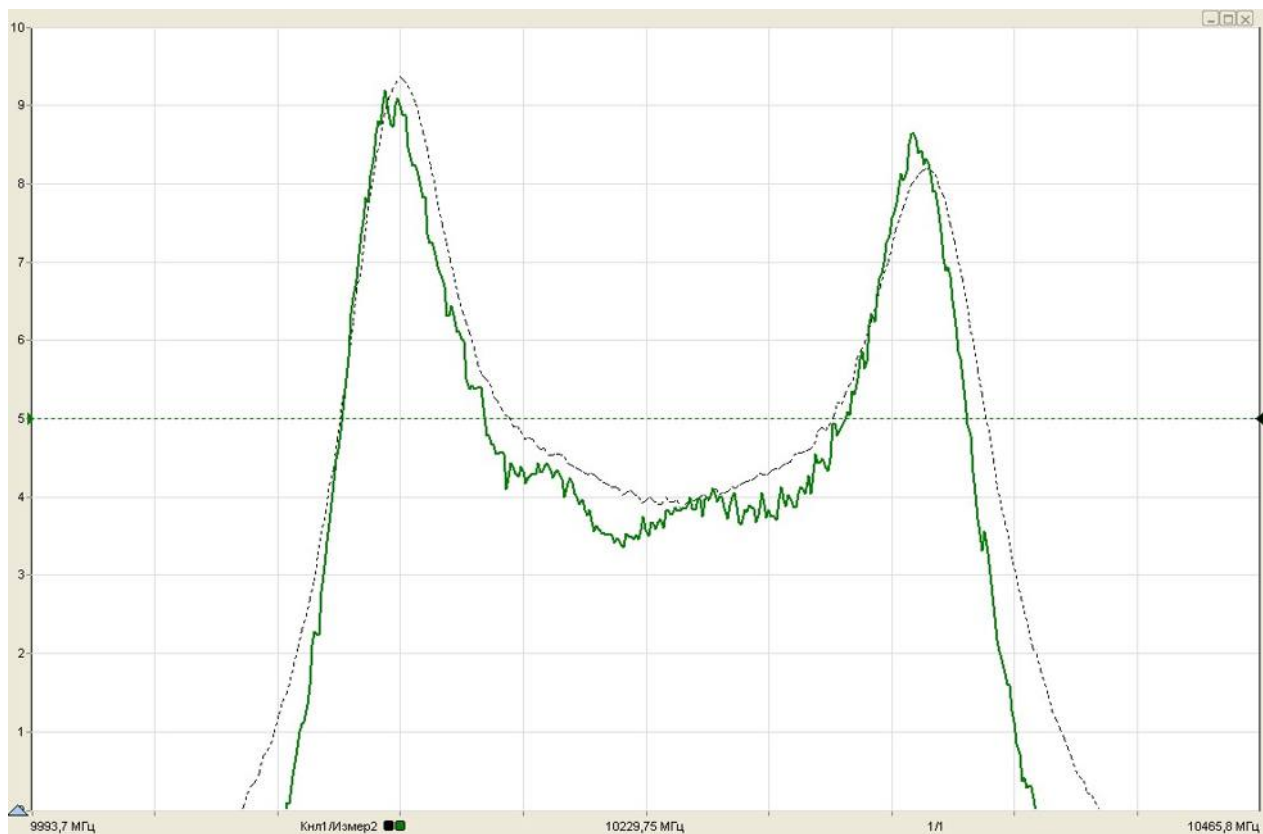
Рисунок 5.32 – Результаты измерений ГВЗ
