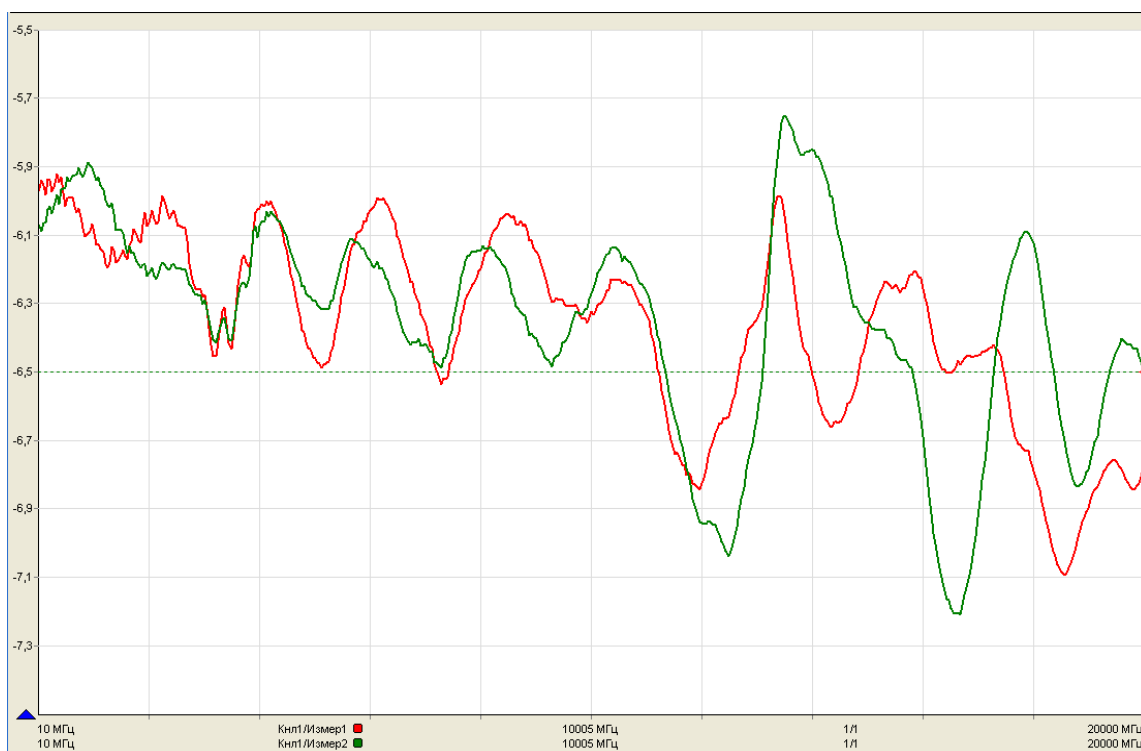
Рисунок 5.12 – Графики измерения модулей КП делителя мощности
