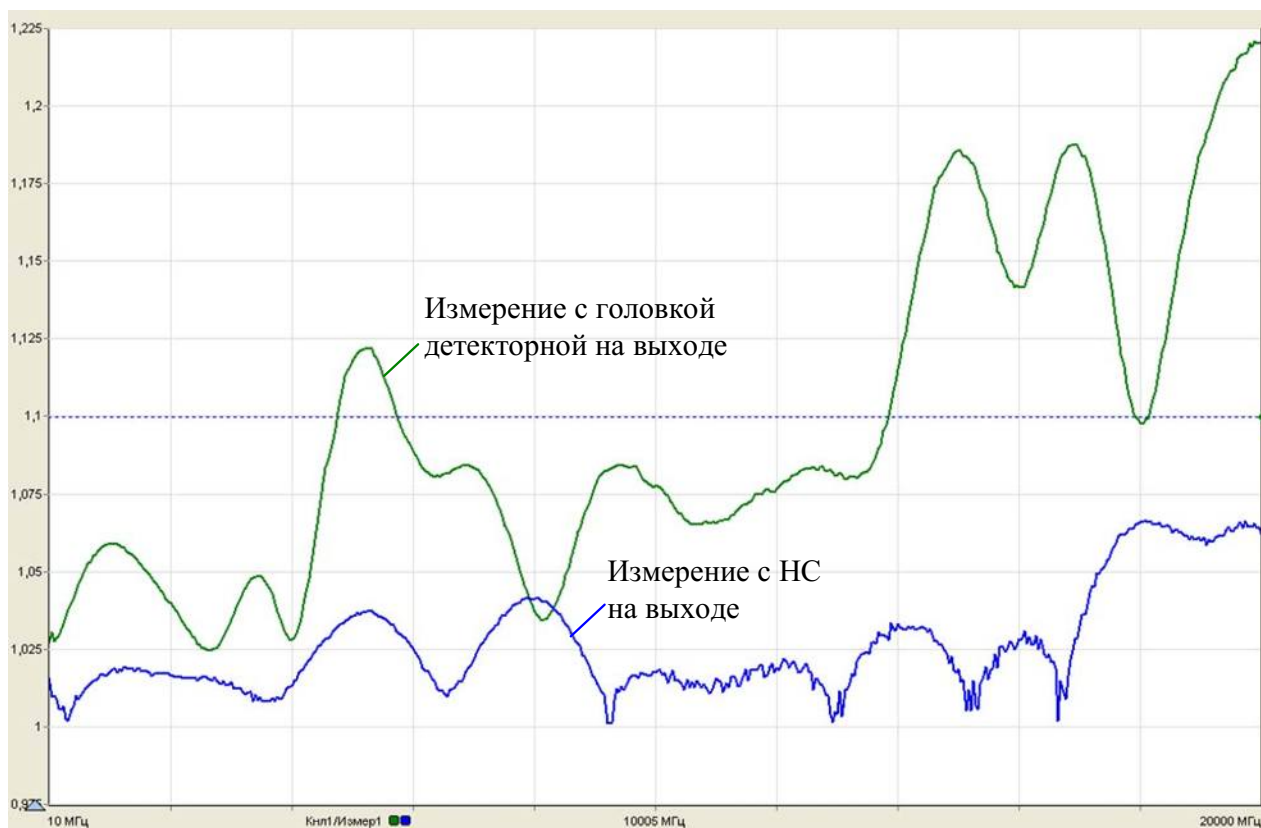
Рисунок 5.20 – Результаты измерений КСВН перехода
