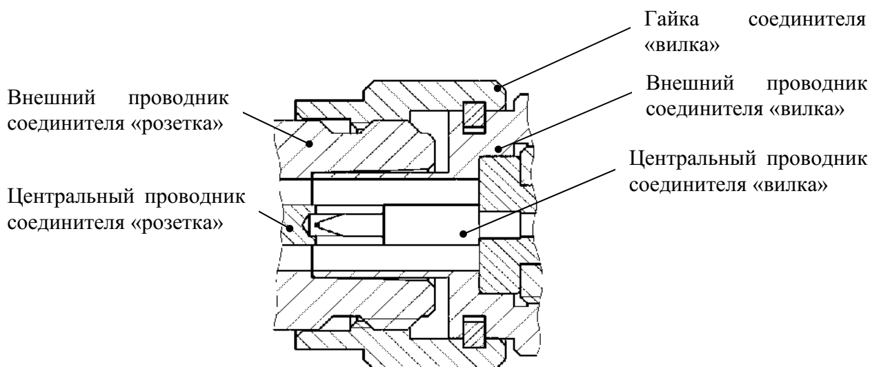
Рисунок 5.1 – Сочленение соединителей типов III или N
