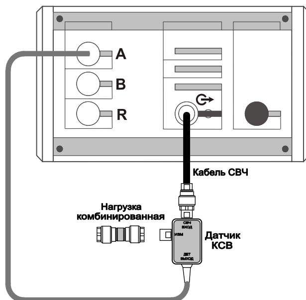
Рисунок 4.5 – Схема калибровки в режиме измерений модуля КО
