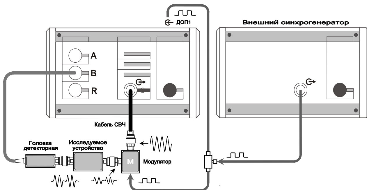
Рисунок 5.37 – Схема измерения модуля КП с внешним синхрогенератором
