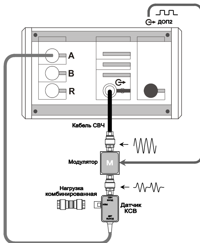
Рисунок 5.34 – Схема калибровки КО с внутренним синхрогенератором
