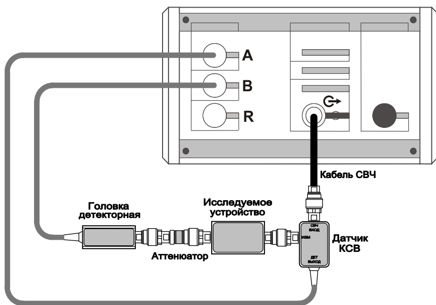
Рисунок 5.23 – Типичная схема измерений модуля КП и КО
