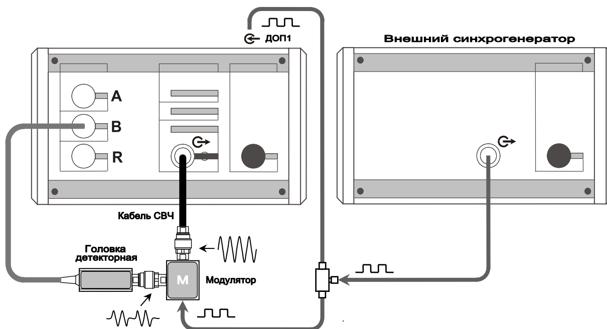
Рисунок 5.36 – Схема калибровки КП с внешним синхрогенератором
