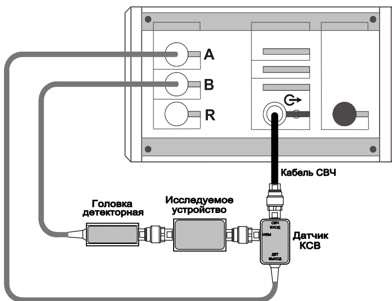
Рисунок 5.22 – Типичная схема измерений модуля КП и КО
