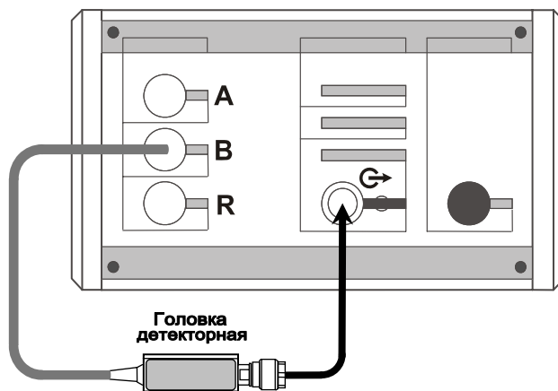
Рисунок 4.7 – Схема измерений мощности
