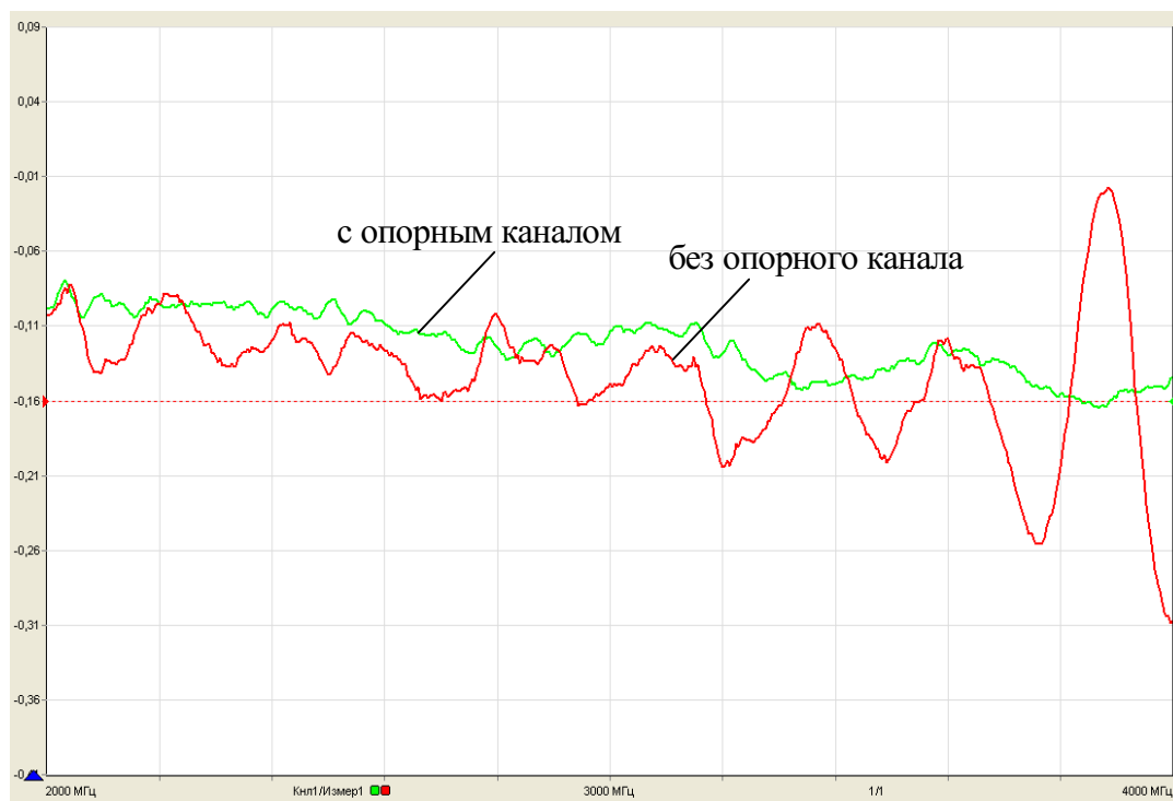
Рисунок 5.9 – Измерение модуля КП кабельной сборки
