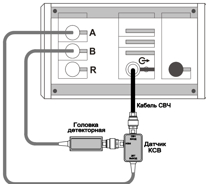
Рисунок 5.21 – Схема калибровки
