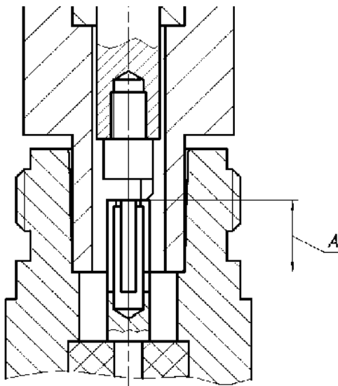
Рисунок 4.3 – Проверка размера «А» соединителя «розетка»
