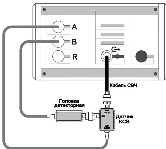
Рисунок 4.6 – Схема калибровки в режиме измерений модуля КП
