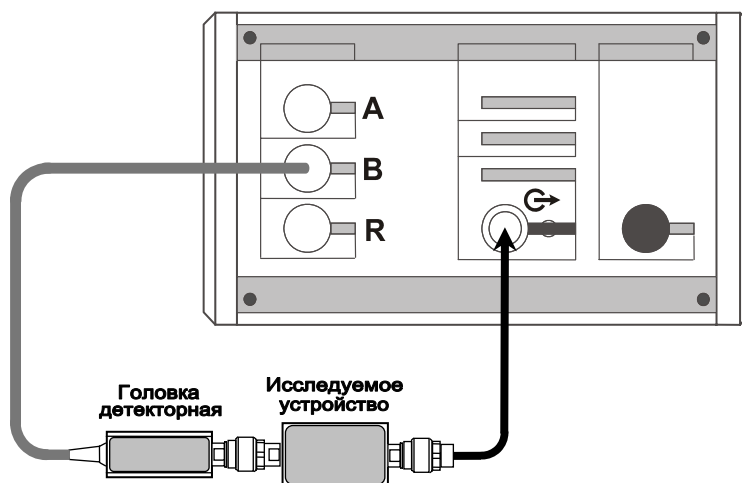
Рисунок 5.5 – Схема измерений мощности на выходе ИУ с внешним сигналом
