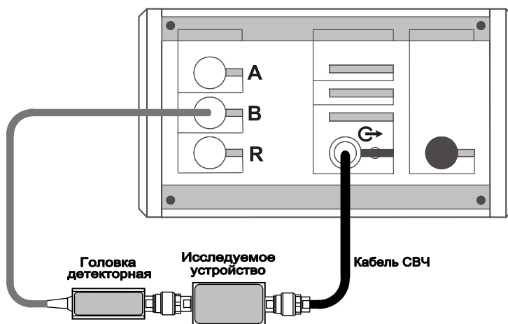
Рисунок 5.30 – Схема измерений
