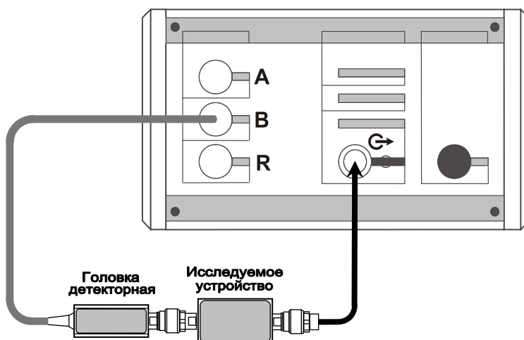
Рисунок 5.6 – Схема измерений модуля КП двухпортовых устройств
