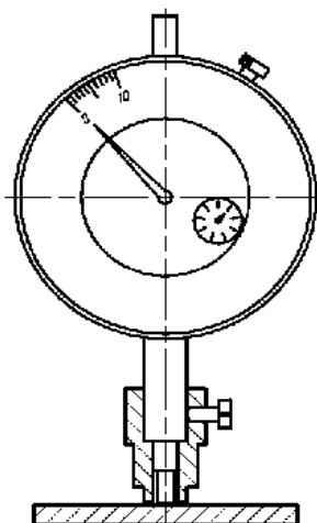
Рисунок 4.2 – Установка нуля
