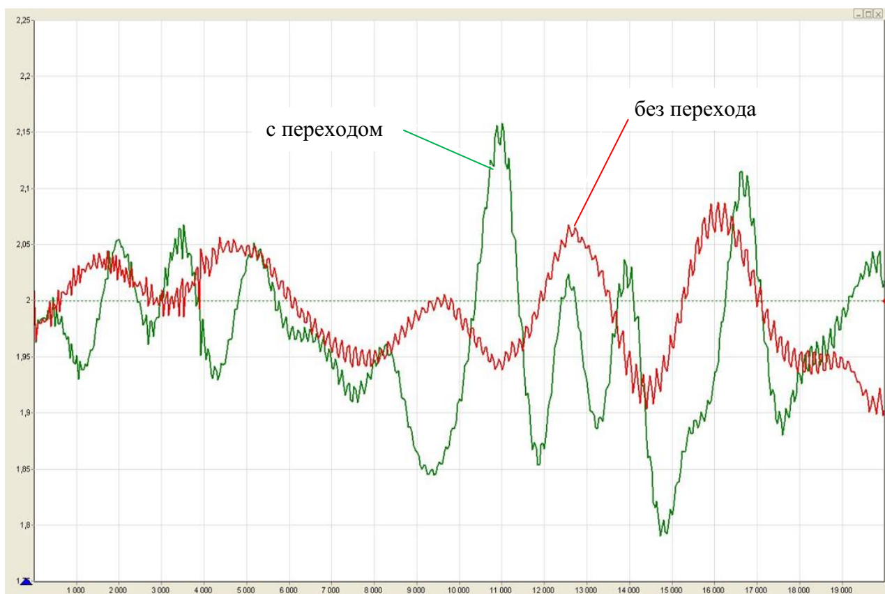
Рисунок 5.18 – Результаты измерений КСВН нагрузки (КСВН = 2,0)
