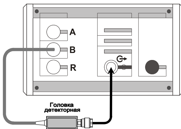
Рисунок 5.31 – Схема калибровки в режиме измерений модуля КП
