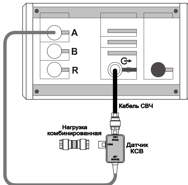
Рисунок 5.38 – Схема калибровки КО
