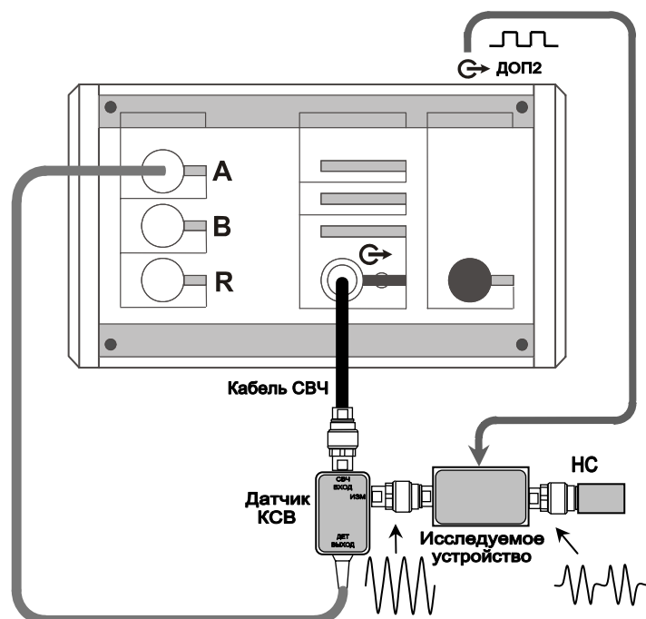
Рисунок 5.39 – Схема измерения модуля КО с внутренним синхрогенератором
