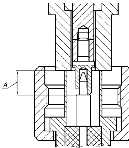
Рисунок 4.4 – Проверка размера «А» соединителя «вилка»
