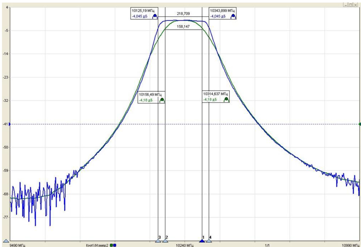
Рисунок 5.8 – График измерения модуля КП полосового фильтра
