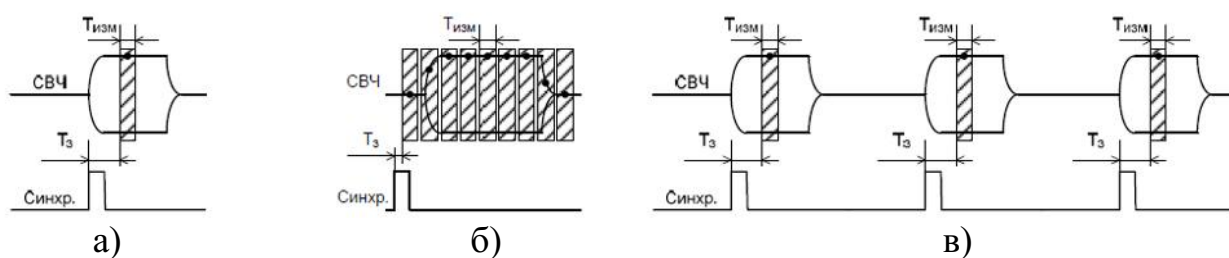
Рисунок 5.33 – Варианты выборки импульса
