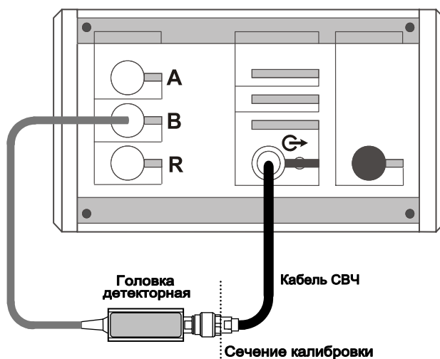
Рисунок 5.7 – Схема калибровки в режиме измерений модуля КП
