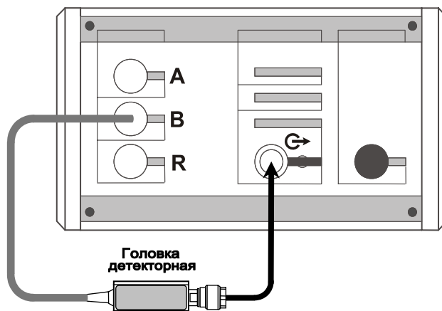
Рисунок 5.40 – Схема калибровки КП с внешним синхрогенератором
