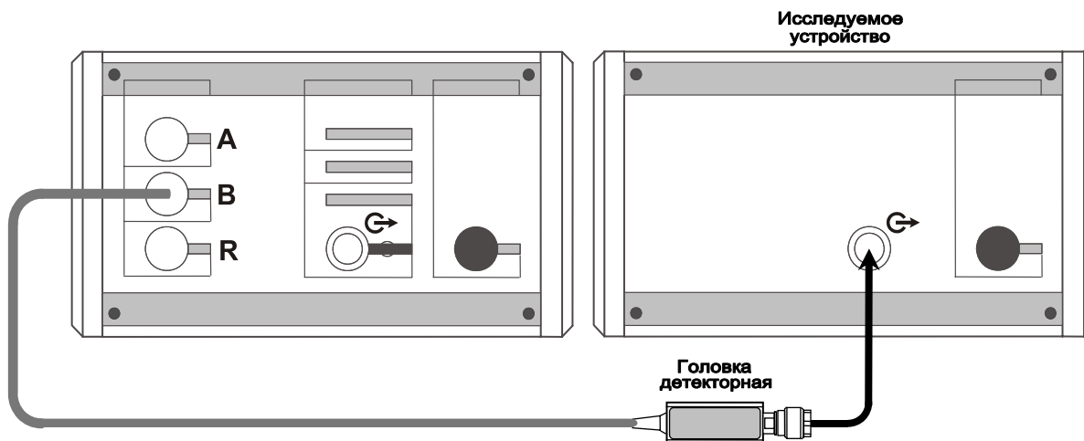
Рисунок 5.4 – Схема измерений мощности на выходе устройств со встроенными источниками сигналов
