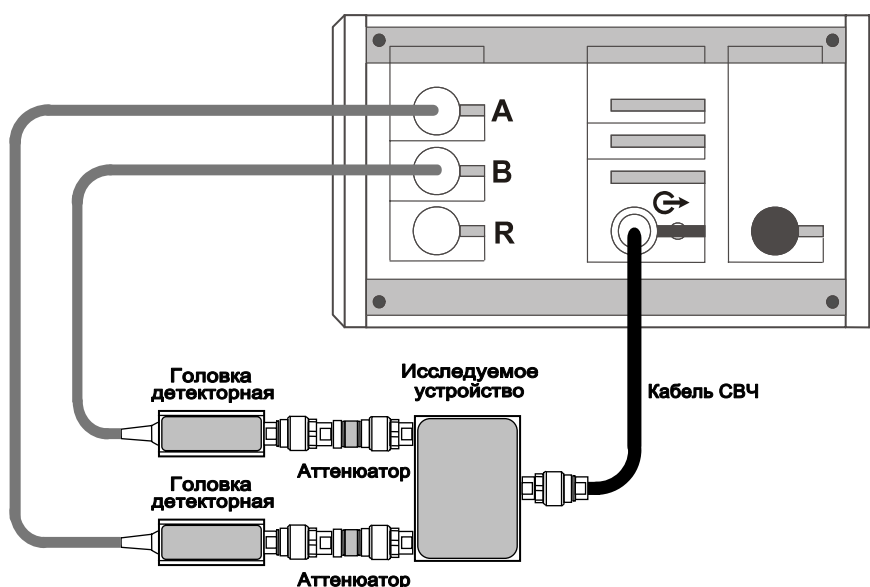
Рисунок 5.11 – Схема измерений модуля КП трехпортовых устройств без преобразования частоты
