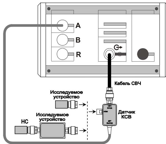
Рисунок 5.17 – Схема измерений модуля КО, КСВН
