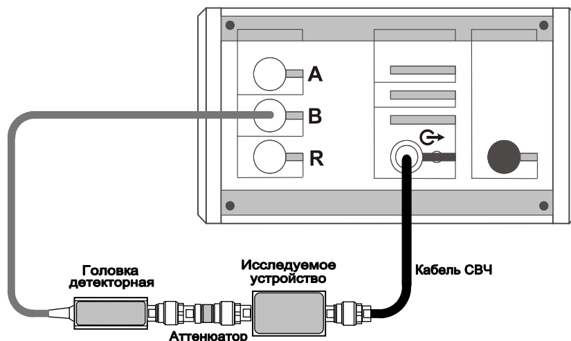
Рисунок 5.25 – Типичная схема измерения динамических характеристик
