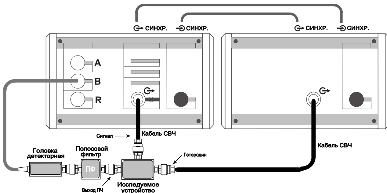
Рисунок 5.13 – Синхронная перестройка частоты сигнала и гетеродина
