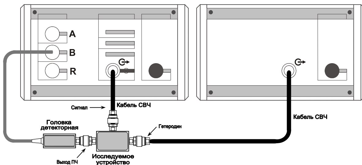
Рисунок 5.14 – Измерение с фиксированной частотой гетеродина
