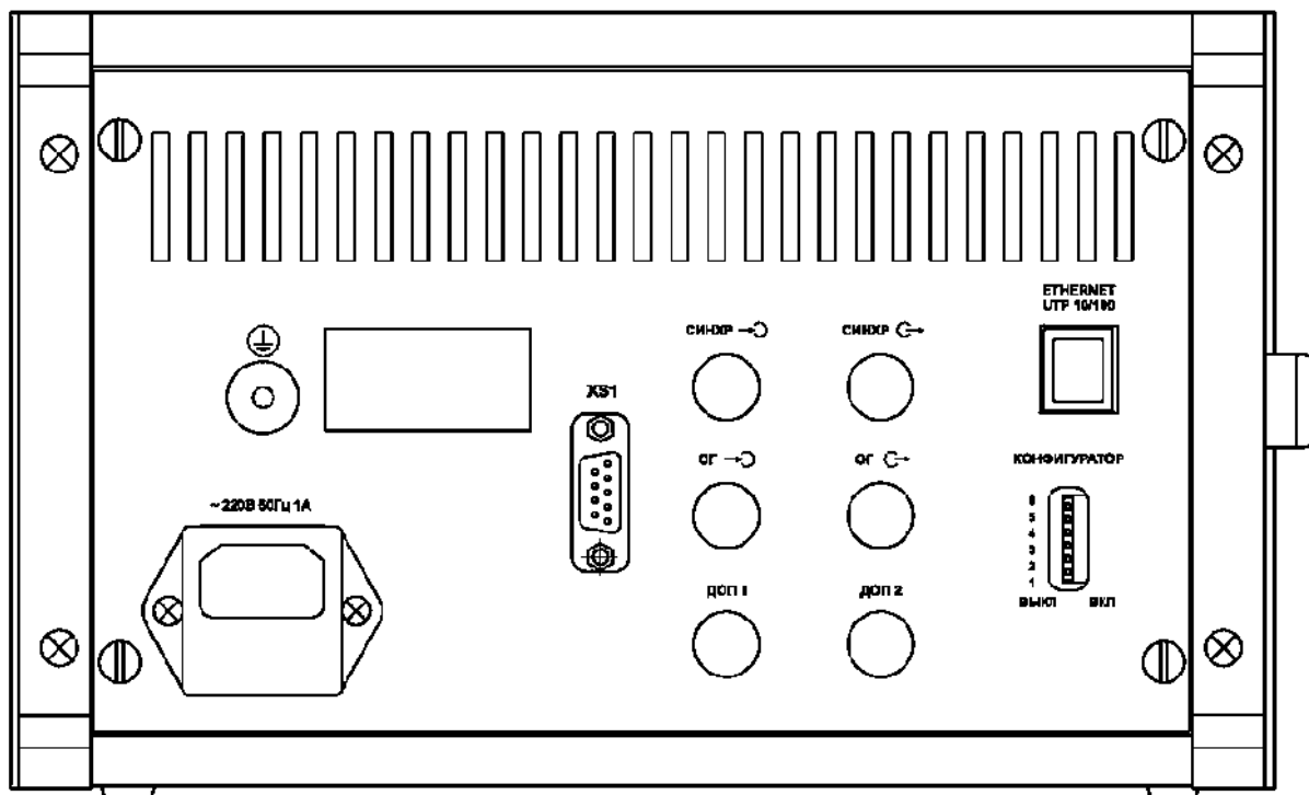
Рисунок 4 – Задняя панель
