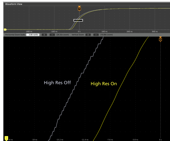
Осциллограф смешанных сигналов серии 6 с 12-разрядным АЦП и режимом High Res обладает лучшим в отрасли разрешением по вертикали.
