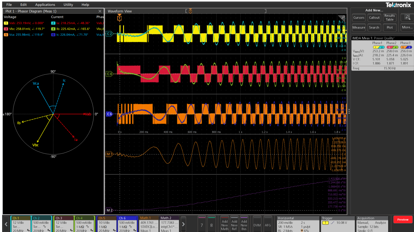
Рис. 31. Слева – векторная диаграмма, отображающая фазу и амплитуду измеренных токов и напряжений трёх фаз питания. В таблице справа показаны все результаты автоматизированных измерений качества питания.
