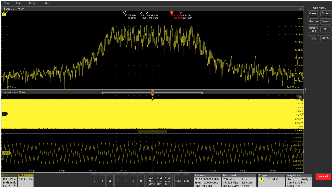
Рис. 27. Нижняя трасса представляет собой график зависимости частоты от времени для сигнала, подаваемого на РЧ вход. Обратите внимание, что индикатор ST расположен в области перехода с низкой частоты на среднюю; таким образом, энергия распределена между несколькими частотами. С помощью графика зависимости частоты от времени можно легко отслеживать различные скачки частоты, что упрощает описание поведения устройства при переключении между частотами.
