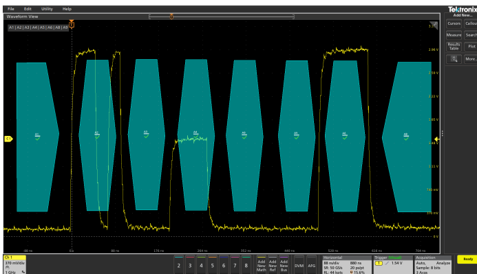
Рис. 14. Зоны визуального запуска изолируют интересующее событие и позволяют экономить время за счет захвата только тех событий, которые вы хотите видеть.
