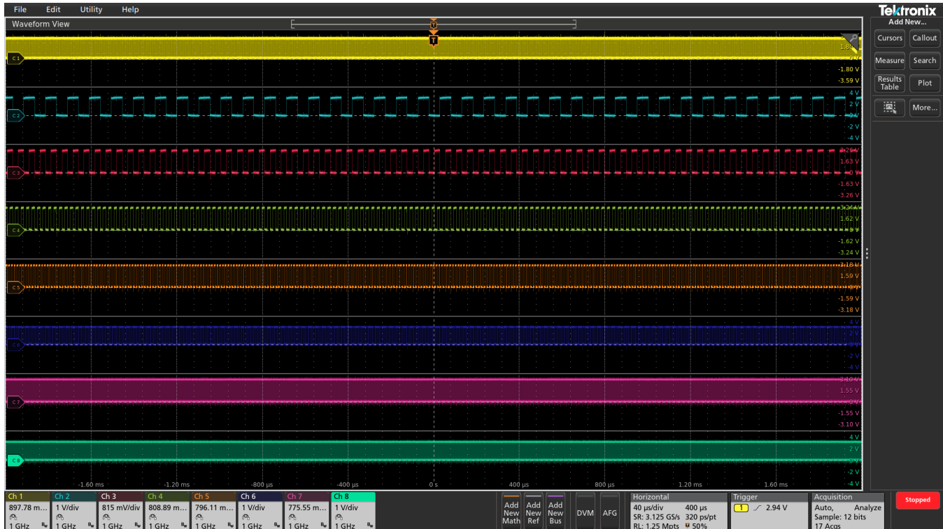
Рис. 5. Режим отображения осциллограмм друг над другом позволяет просматривать их одновременно при максимальном использовании разрешения АЦП по каждому входу, что обеспечивает наиболее точное измерение.
