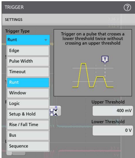
Рис. 13. Большое число функций запуска и контекстно-зависимая справочная система в меню запуска позволяют быстро выделить интересующее событие.
