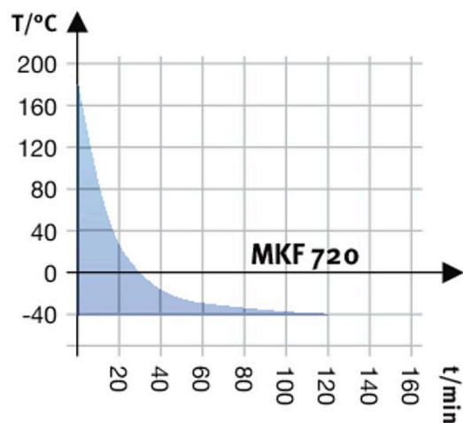
Кривая охлаждения
