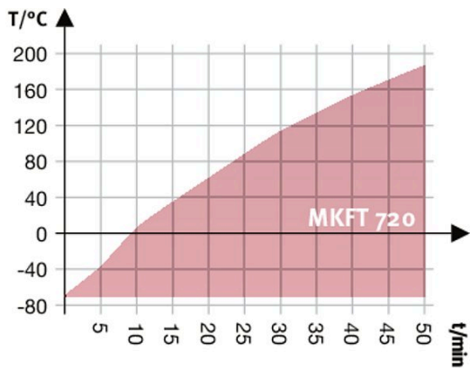
Кривая нагрева
