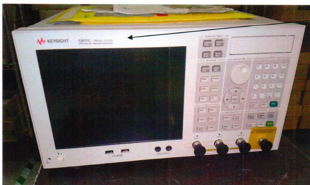
а) Место для нанесения знака утверждения типа Рисунок 1 – Внешний вид. Вид спереди
