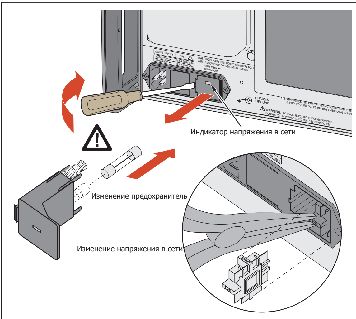
Рисунок 7-1. Извлечение предохранителя
