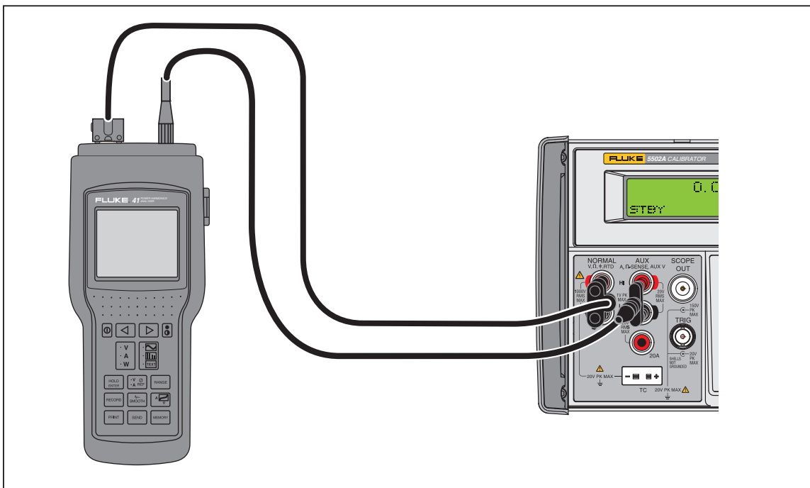
Рисунок 4-18. Подключения кабелей для тестирования функции измерения в ваттах для устройств серии 40 gvx028.eps
