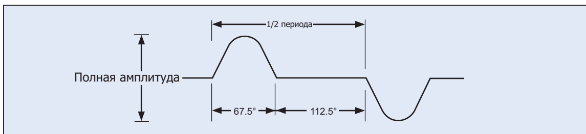
Рисунок 4-14. Усеченная синусоида
