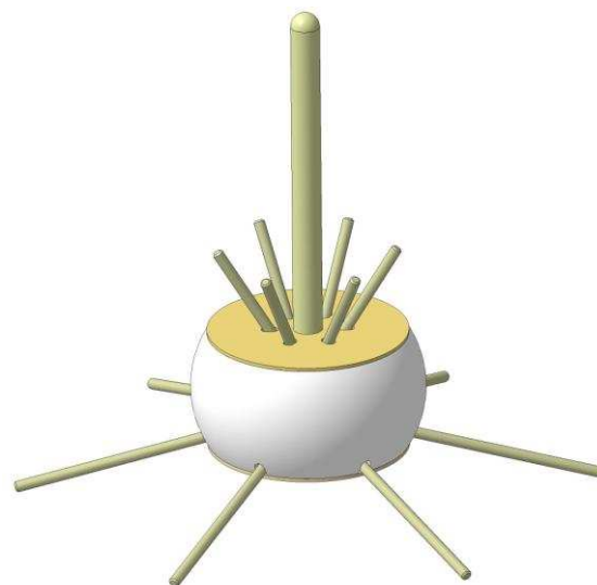
Рис.2 3D модель антенны АС7.22
