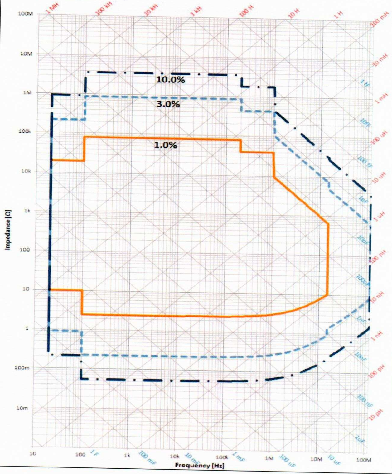
График погрешности измерения импеданса у 3,5-миллиметрового порта импедансного пробника 42941А, присоединенного к прибору E4990A (уровень сигнала генератора 0,5 Вскз, время измерения – 5 с)
