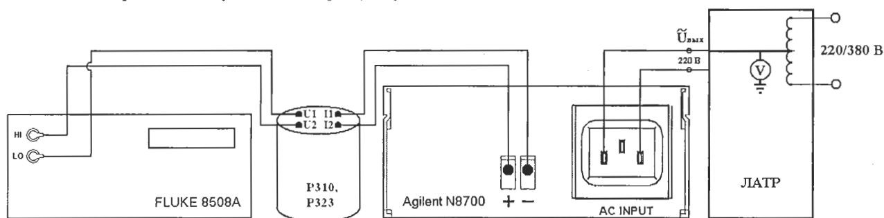
Рисунок 3 Структурная схема соединения приборов для определения погрешности установки силы постоянного тока и нестабильности силы постоянного тока на выходе при изменении напряжения электропитания источника.
