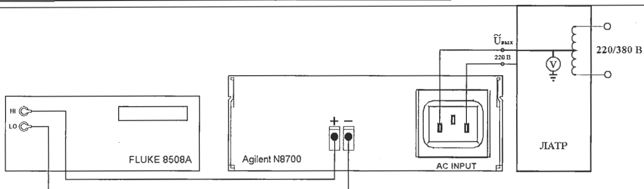
Рисунок 1 Структурная схема соединения приборов для определения абсолютной погрешности установки напряжения постоянного тока, определения нестабильности напряжения постоянного тока на выходе при изменении напряжения электропитания источника.
