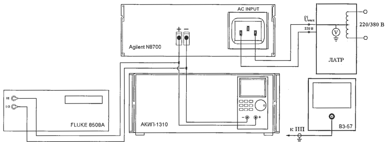
Рисунок 2 Структурная схема соединения приборов для определения нестабильности напряжения постоянного тока на выходе при изменении силы тока в нагрузке, уровня пульсаций напряжения постоянного тока на выходе.
