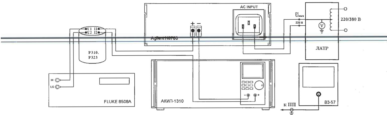
Рисунок 4 Структурная схема соединения приборов для определения нестабильности силы постоянного тока на выходе при изменении напряжения на нагрузке, уровня пульсаций силы постоянного тока на выходе.
