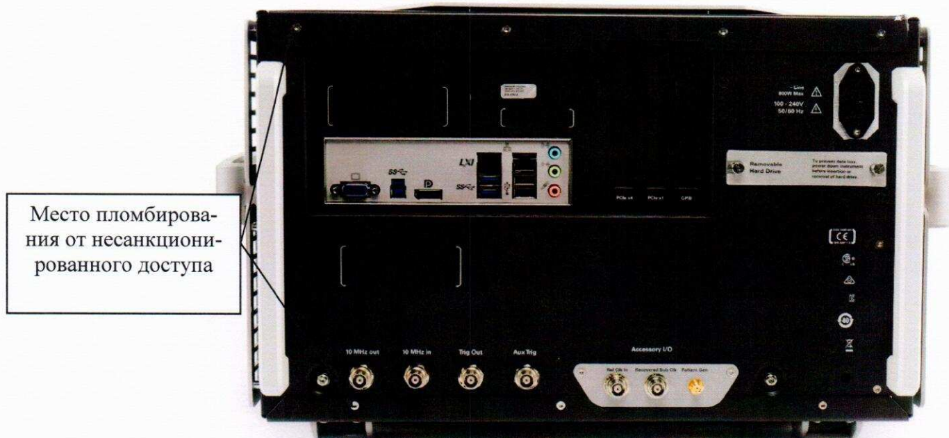
Рисунок 2 - Схема пломбировки от несанкционированного доступа
