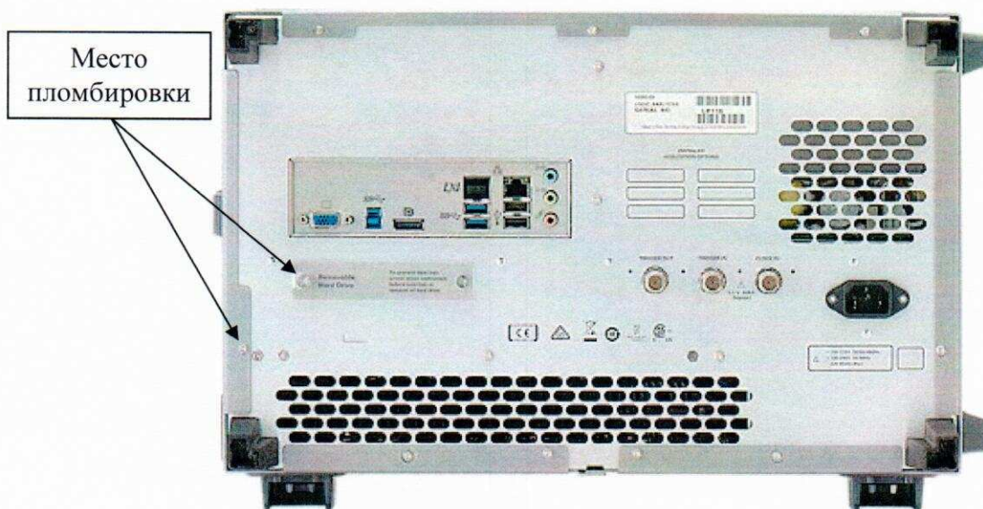
Рисунок 2 - Общий вид анализаторов 16861А, 16862А, 16863А, 16864А (задняя панель)
