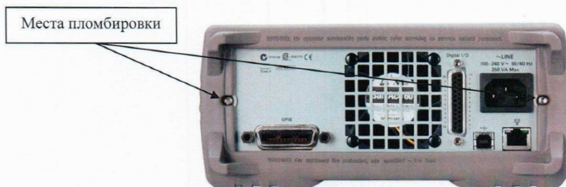
Рисунок 2 – Внешний вид задней панели источников-измерителей B2901A, B2911A
