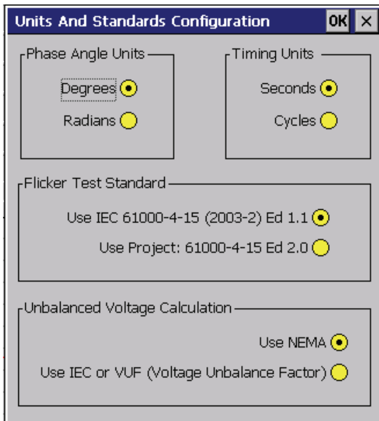
Рис. 4-5. Units and Standards Configuration (Конфигурация единиц и стандартов)
