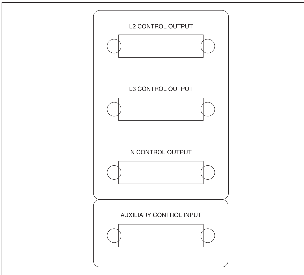
Рис. 2-1. Разъемы вспомогательных устройств на задней панели 6105A
