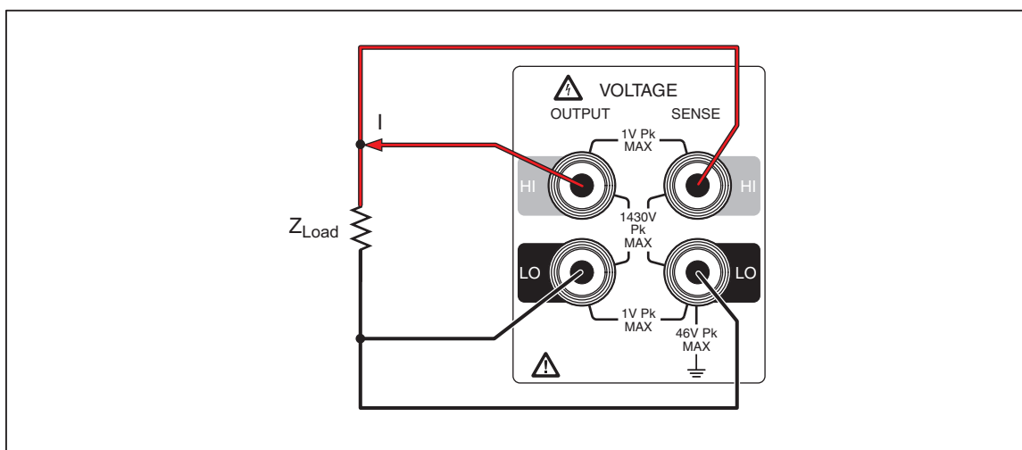
Рис. 3-10. Четырехпроводная измерительная схема
