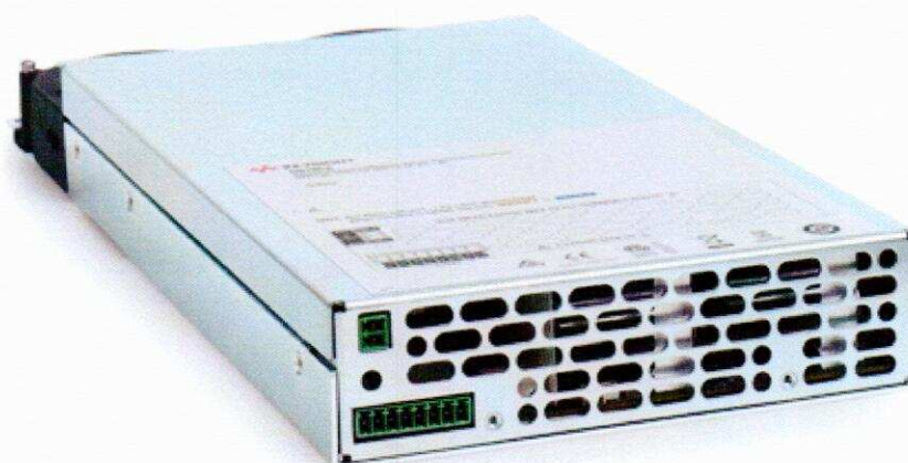
Сменные модули N6785A, N6786A
