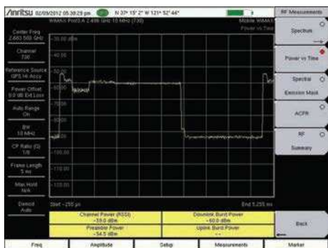
Сигнал WiMAX
