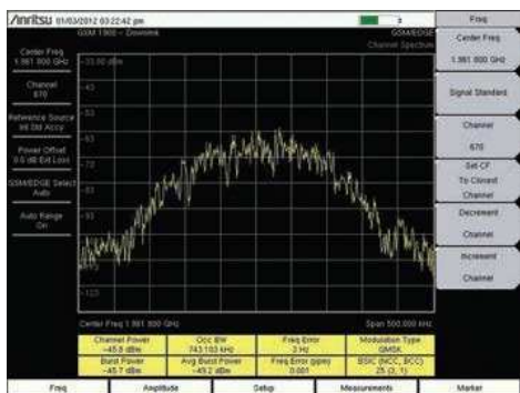
Сигнал GSM
