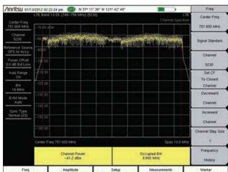
Сигнал LTE
