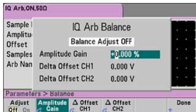
Рис. 4. Экран настройки баланса IQ
