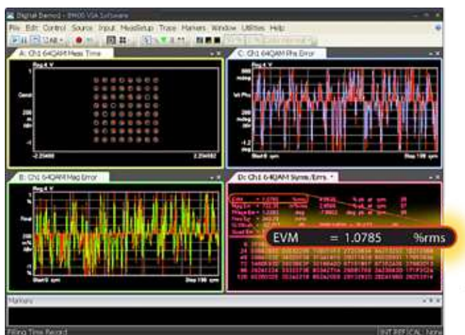
Рис. 5. Сигнальное созвездие и амплитуда вектора ошибки модулирующего сигнала 64-QAM с добавленным шумом.
