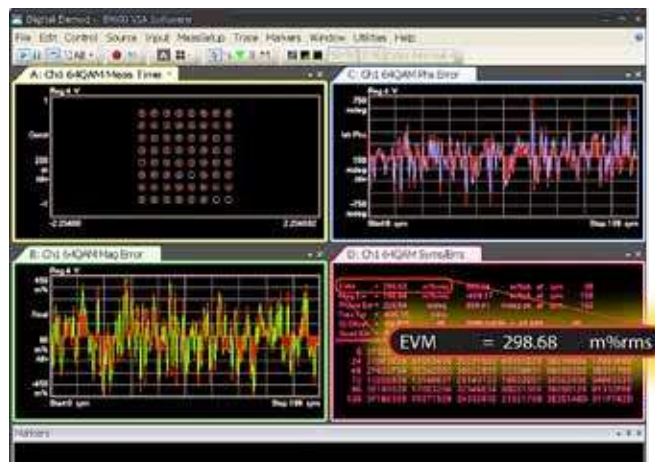
Рис. 3. Сигнальное созвездие и амплитуда вектора ошибки модулирующего сигнала 64-QAM
