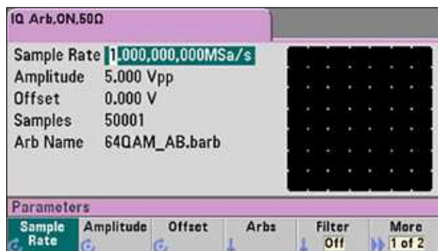
Рис. 2. Снимок экрана плеера IQ-сигналов 33500В
