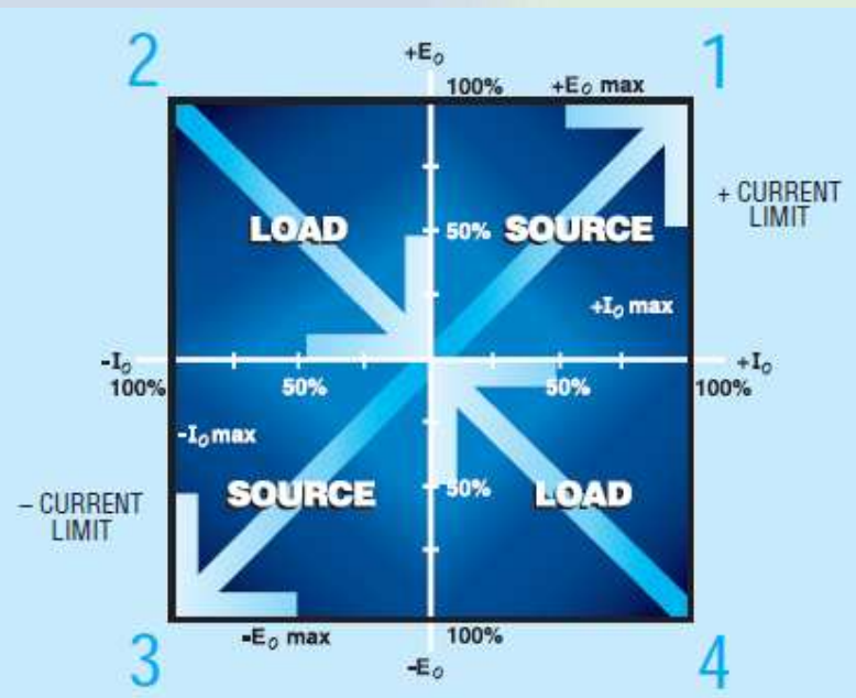
напряжение E_o и протекающий в данной цепи ток I_o
