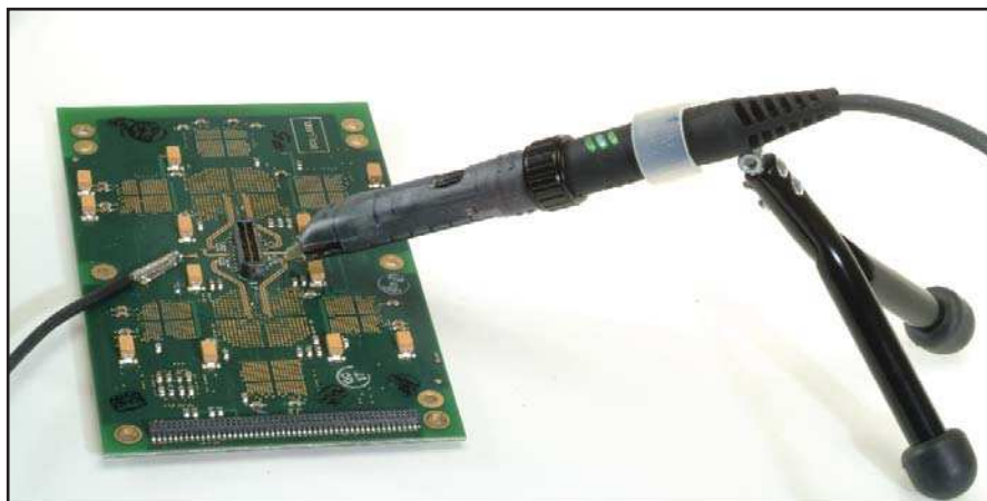
Пробник WaveLink с регулировкой TwinTips в держателе "FreeHand"
