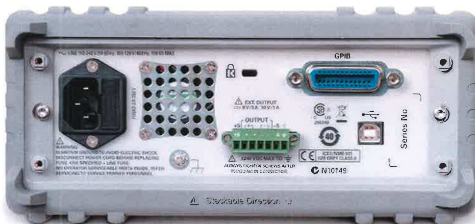
Рисунок 2 – Общий вид мультиметров цифровых/источников питания U3606B. Задняя панель
