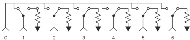
СХЕМА ПОЛОЖЕНИЙ ПЕРЕКЛЮЧАТЕЛЯ
