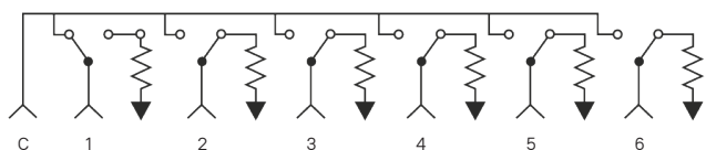
СХЕМА ПОЛОЖЕНИЙ ПЕРЕКЛЮЧАТЕЛЯ
