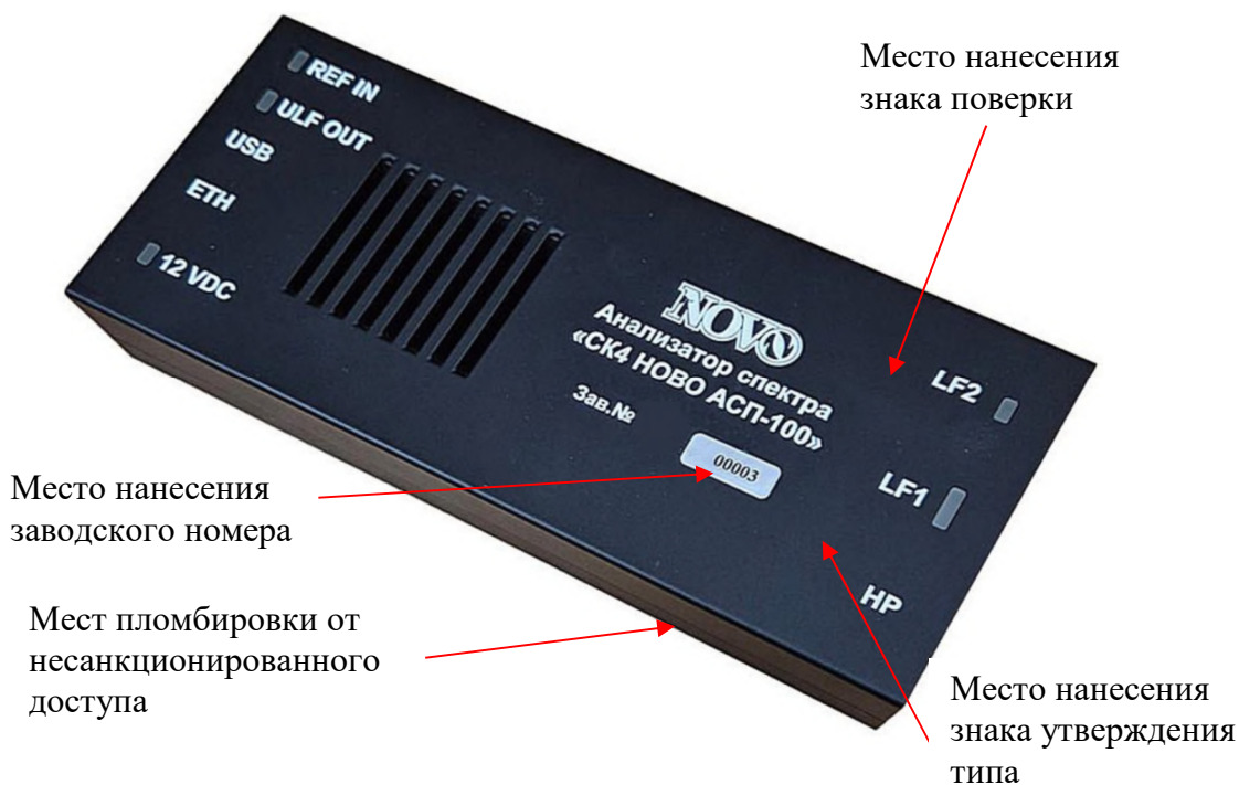
Рисунок 1 – Общий вид анализатора
