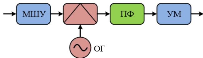
Активный ретранслятор
