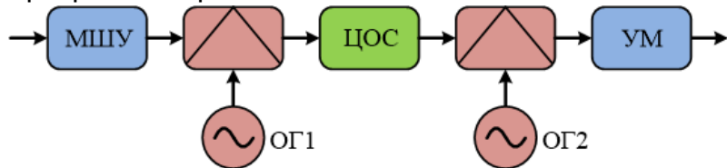
Регенеративный ретранслятор
