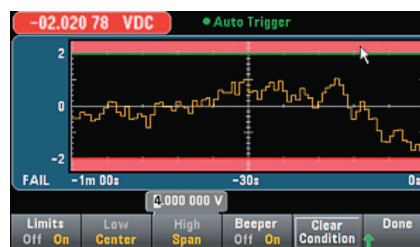
Рисунок 8. Пример допусковых испытаний с графиком тренда.
