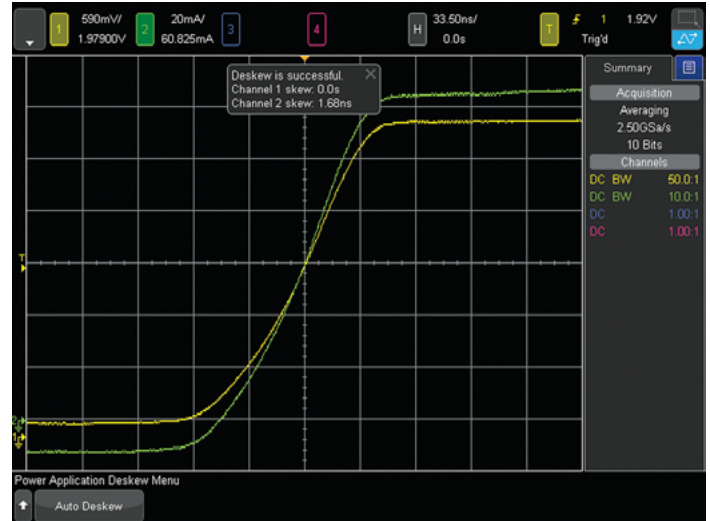
Рис. 13. Для получения точных результатов измерения параметров мощности крайне важно скомпенсировать временную задержку между пробниками напряжения и токовыми пробниками.
