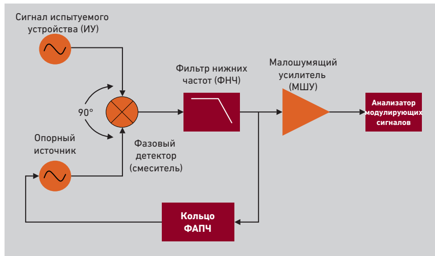
Рисунок 4 - В этом методе используются опорный источник и двойной балансный смеситель в качестве основы фазового детектора.
