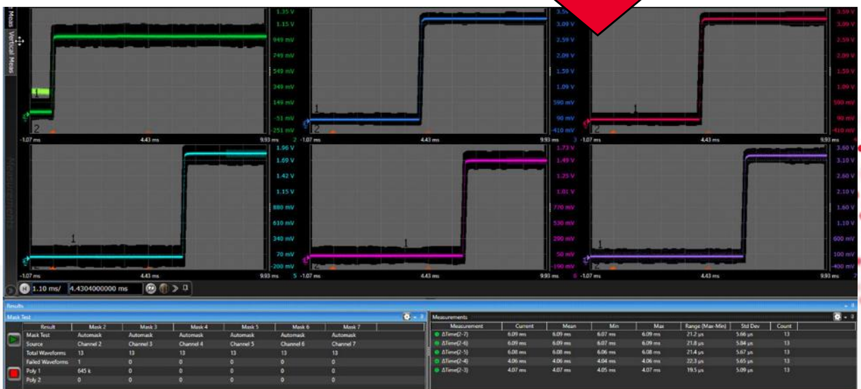
Благодаря разделению сигналов по различным шкалам и возможности независимого тестирования по маске на каждом канале можно непрерывно тестировать эти шесть шин питания в течение тысяч циклов запуска.
