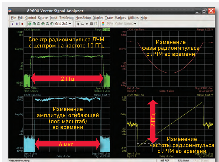
Рисунок 3 - Здесь показан пример измерения характеристик широкополосного радиои́мпульса с ЛЧМ РЛС с использованием программного обеспечения векторного анализа сигналов в осциллографе 90000X.
