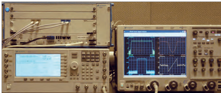
Рисунок 1: Здесь показана типичная испытательная установка, используемая для создания и анализа широкополосных сигналов РЛС и систем спутниковой связи. Широкополосный генератор сигналов произвольной формы показан слева сверху, генератор сигналов серии PSG с широкополосными I/Q входами - слева внизу, а широкополосный осциллограф серии 90000X с программным обеспечением векторного анализа сигналов - справа
