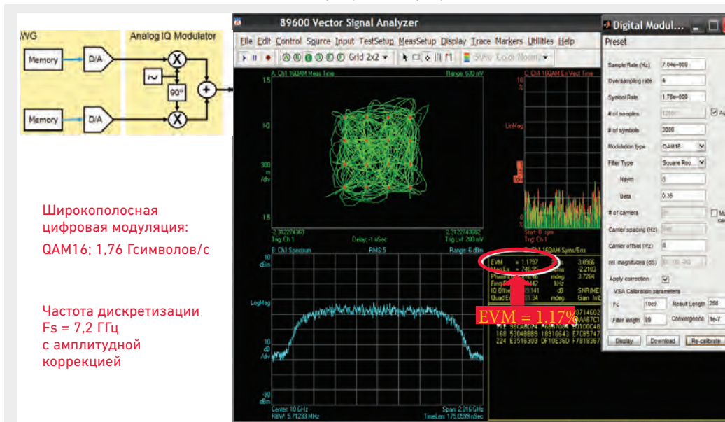
Рисунок 4 – В четырёх квадрантах дисплея программы векторного анализа сигналов (VSA) показаны: звёздная диаграмма (слева сверху), спектр сигнала X-диапазона (10 ГГц) (слева снизу), зависимость EVM от времени (справа сверху) и итоговое значение EVM (справа снизу). В данном примере остаточное значение EVM получено в результате объединения генератора СПФ, генератора сигналов серии PSG с широкополосными I/Q входами и цифрового осциллографа с полосой пропускания 32 ГГц.
