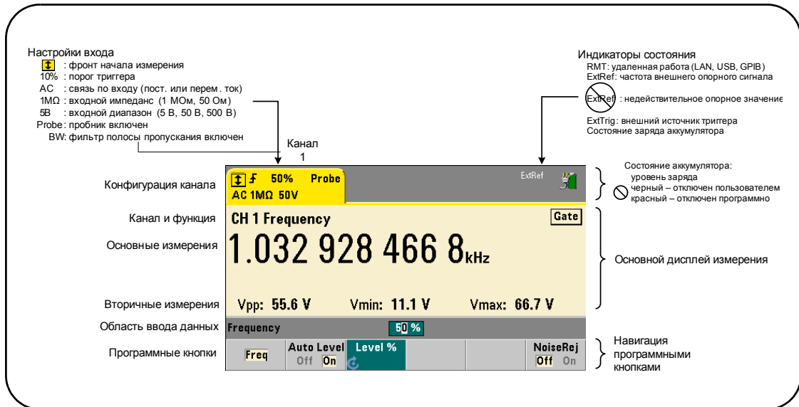
Рисунок 1-2 Дисплей 53210A
