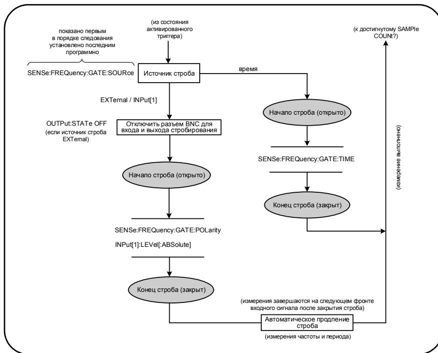
Рисунок 5-5 Последовательность настройки источника строба
