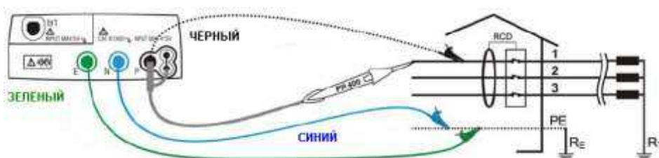
• Рис.23: Подключение прибора для измерения полного сопротивления петли P-PE в трехфазной сети 400В + PE (no N) при помощи измерительных проводов или опционального щупа-пробника
