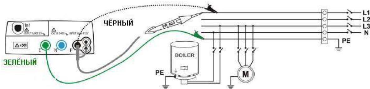
Рис.8: Прибор подключен к сети при помощи отдельных измерительных проводов и опционального щуп-пробника
